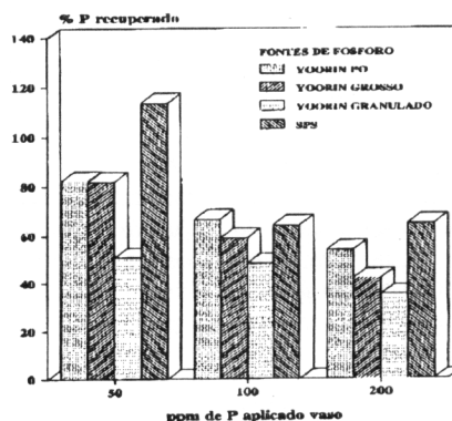
Figura 1- Fósforo (%) extraído nos sete cultivos em função de diferentes fontes, granulometrias e níveis .
