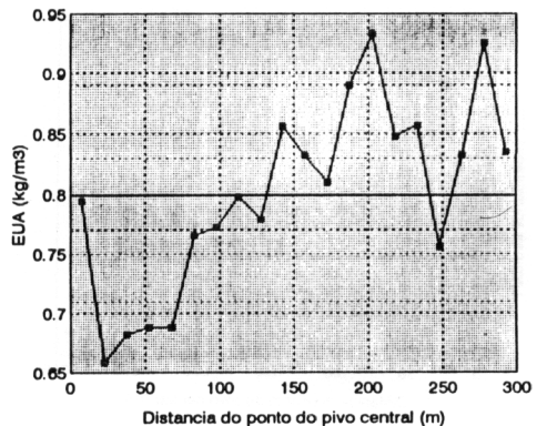
Figura 4 - Eficiência de uso da água (EUA) ao longo do raio do pivô.
