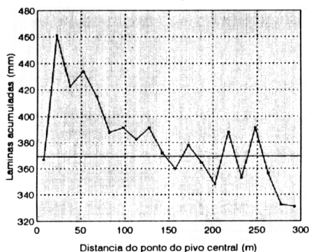
Figura 1 - Distribuição das lâminas acumuladas (16 irrigações) ao longo do raio do pivô.
