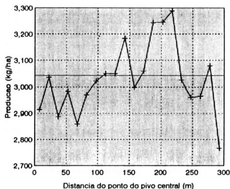
Figura 2 - Produção da cultura de feijão irrigado, ao longo do raio do pivô.
