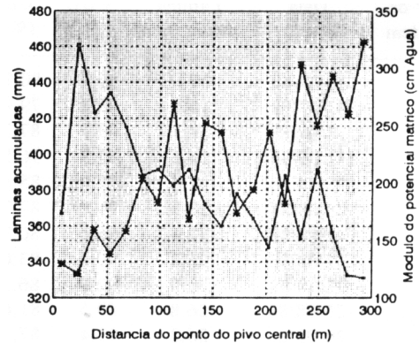
Figura 3 - Potencial mátrico (cm água) e lâmina de água aplicada (16 irrigações) ao longo do raio do pivô.
