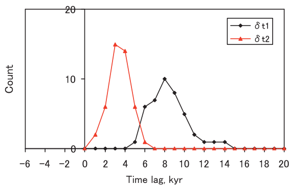
図7 入射熱の変化に対する氷床体積の変動の時間遅れのヒストグラム 計算条件：氷床体積の最大しきい値 V_{max} = 46 \times 10^6 \text{km}^3 、最小しきい値 V_{min} = 3 \times 10^6 \text{km}^3 、氷床体積の堆積容量 R=10\text{Sv} \cdot \text{kyr} 、3000kyr 間の計算
