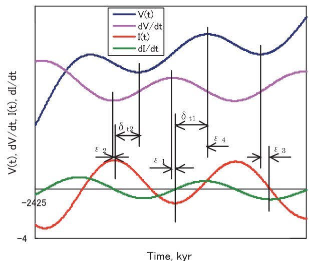
図 5 氷床体積 V(t) 変動とその微分形 dV/dt および入射熱変動 I(t) とその微分形 dI/dt を時間軸上で示した模式図
