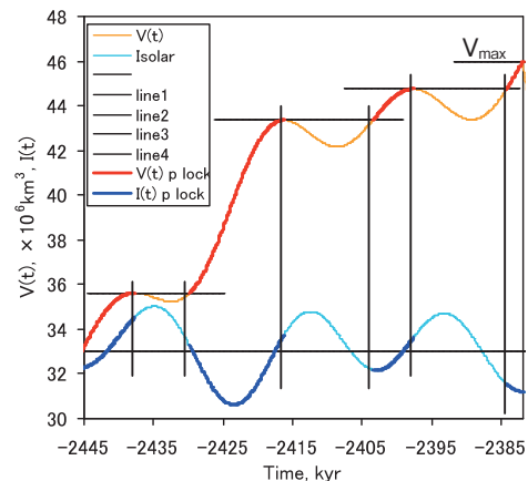
図8 氷床体積の変動におけるターミネーションのタイミング；入射熱のスケールは任意 計算条件：氷床体積の最大しきい値 V_{max} = 46 \times 10^6 \text{km}^3 、最小しきい値 V_{min} = 3 \times 10^6 \text{km}^3 、氷床体積の堆積容量 R=10\text{Sv} \cdot \text{kyr}
