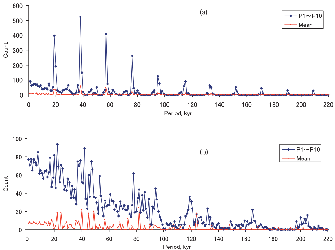
図3 氷期振動 P1～P10 周期のヒストグラム
