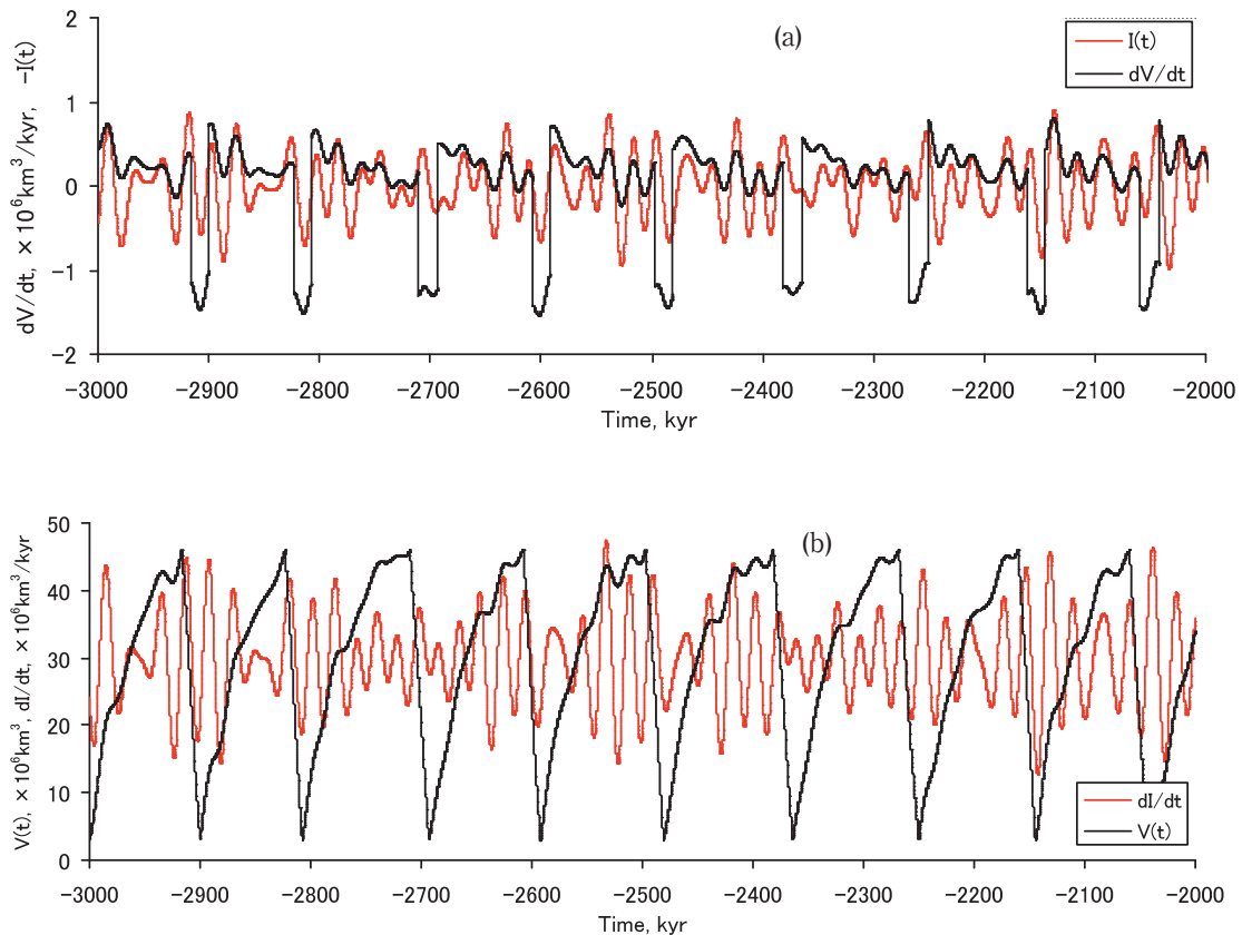
図4 氷床体積 V(t) およびその微分形 dV/dt と入射熱 I(t) とその微分形 dI/dt の時間軸上での変化 計算条件：氷床体積の最大しきい値 V_{max} = 46 \times 10^6 \text{km}^3 、最小しきい値 V_{min} = 3 \times 10^6 \text{km}^3 、氷床体積の堆積容量 R=10Sv \cdot \text{kyr} 、1000kyr 間の計算 (a) 氷床体積の微分形 dV/dt と入射熱 I(t) の変化； dV/dt の単位は任意 (b) 氷床体積 V(t) と入射熱の微分形 dI/dt の変化； dI/dt の単位は任意
