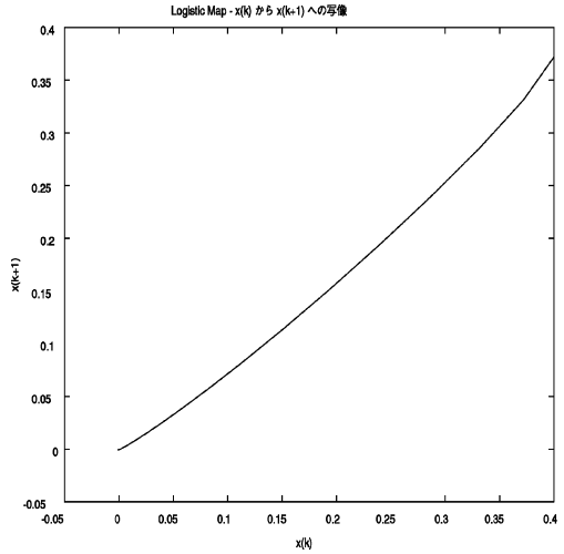
図5 制御過程の写像 x(k) \rightarrow x(k+1) (不動点 x_f=0 )
