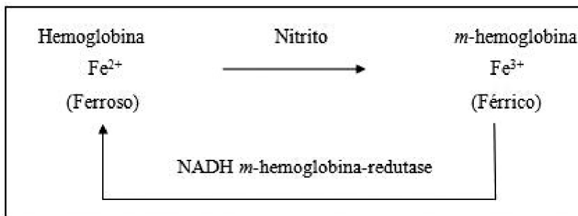
Figura 1. Formação de m -hemoglobina pelo nitrito e sua conversão à hemoglobina.
