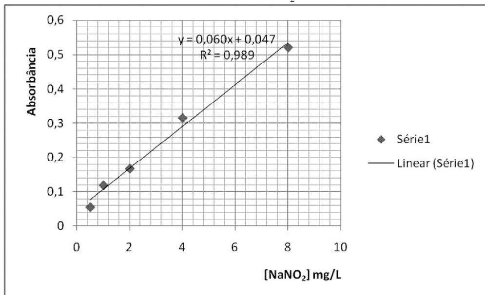
Figura 3. Gráfico de Absorbância em função da concentração de \text{NaNO}_2 , no intervalo entre 0,5 – 8,0 mg/L.
