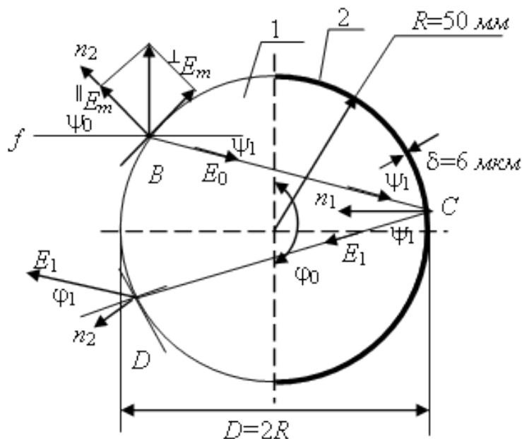
Рис. 1. Прохождение луча в сферической линзе Люнеберга Fig. 1. Passing of a beam in a spherical lens of Lyueneberg
