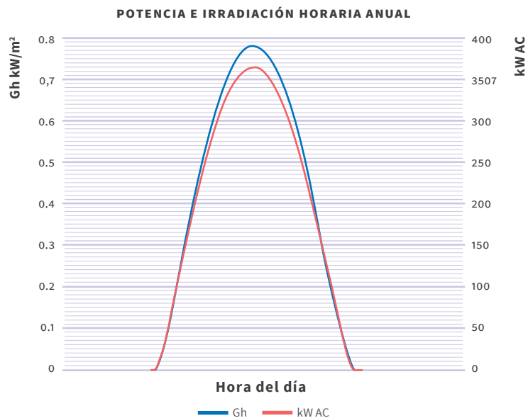
[ Figura 2. Potencia e irradiación horaria anual. ]
