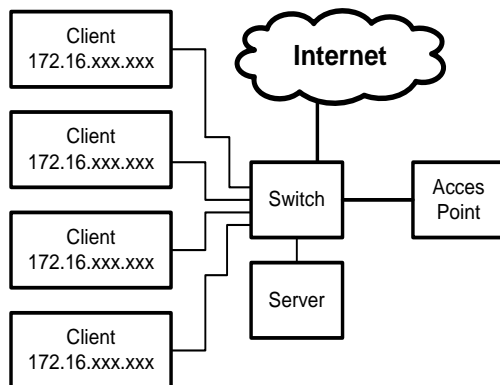
Gambar3. Topologi Jaringan Berjalan
