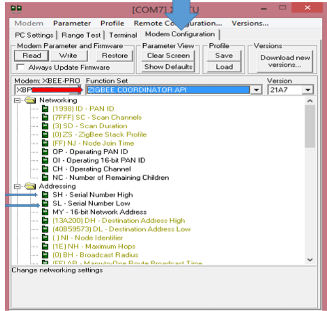
Fig. 10. Configurando Xbee.
