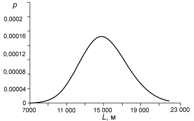
Рис. 3. Функция распределения вероятности p длины L , м, ледника Ханс в стационарных условиях Fig. 3. Probability distribution function p of the Hansreen length L , m, in stationary conditions
