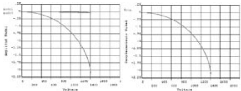
Figura 5. Barrido DC. Contribución de cada modo (izquierda), Deflexión total de la micro-viga (derecha)
