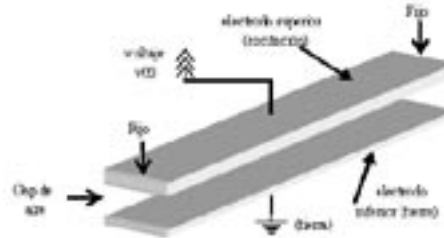
Figura 3. Micro-Viga Electrostática
