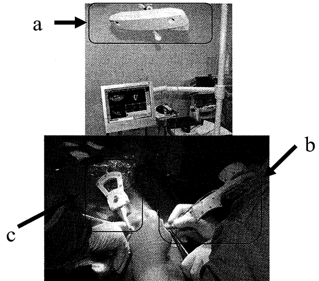
図8 本体とリファレンスポダイ・ハンドピースの位置関係 a: 赤外線カメラ b: レファレンスポダイ c: ハンドピースに接続したLED
