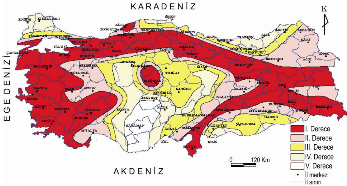
Şekil 4. Deprem şiddetine (derecesine) göre Türkiye deprem bölgelerinin dağılışı (Özmen, vd., (1997)' ne göre yeniden düzenlendi).
