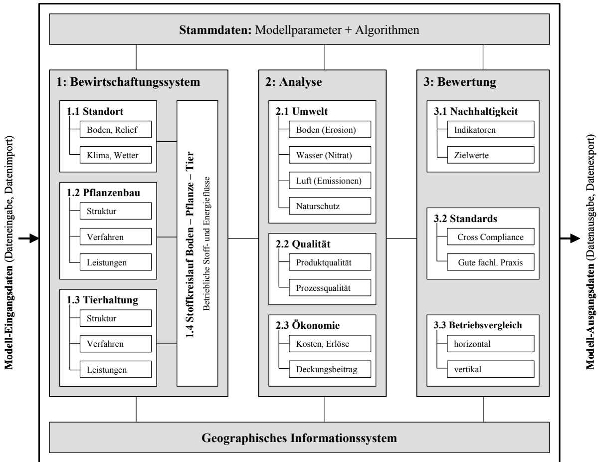
Abbildung 4: Aufbau des Programms REPRO
