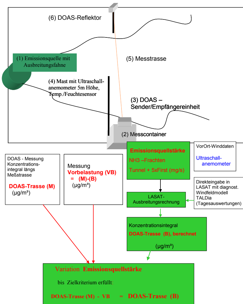
Abbildung 13: Prinzip der Quellstärkenbestimmung diffuser Emissionsquellen mittels DOAS-Trassenmessung und Rückrechnung mit Ausbreitungsmodell LASAT
