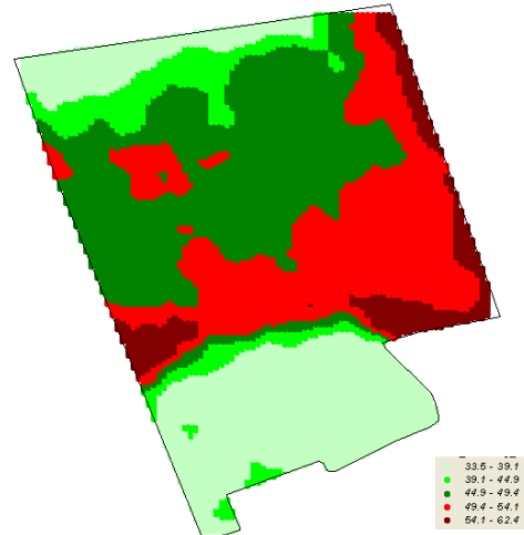
Abbildung 52: Karte der scheinbaren elektrischen Leitfähigkeit (EM38) vom Schlag „Oberweg“
