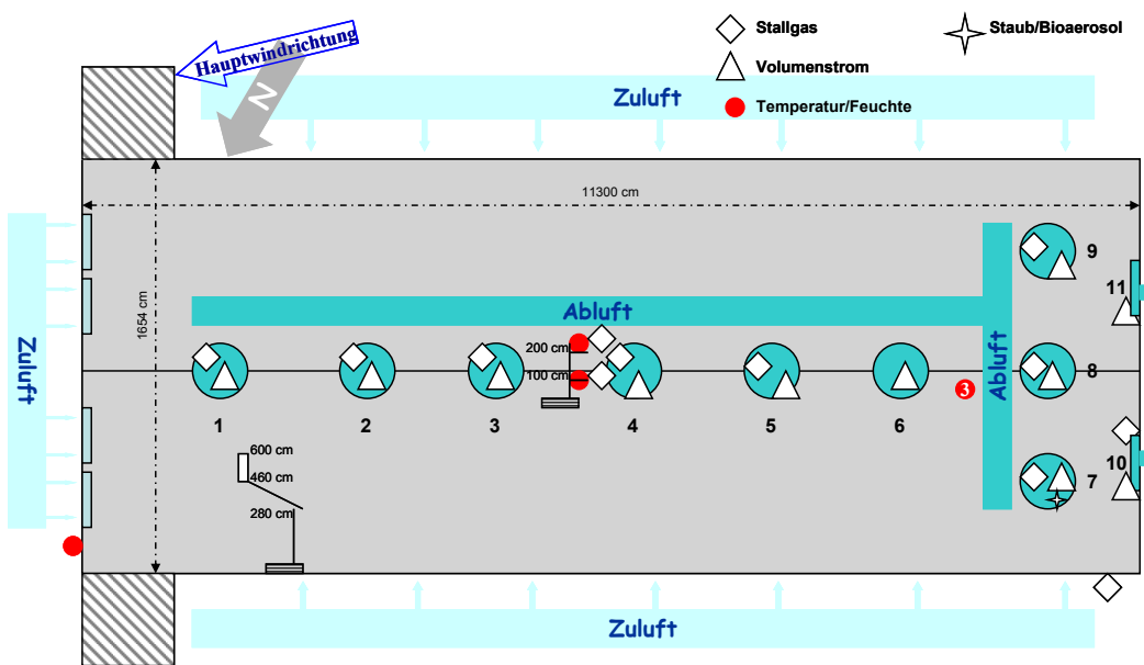
Abbildung 3: Messpunkteplan in der Kleingruppenhaltung KG-2 (> 15.000 Tpl.)
