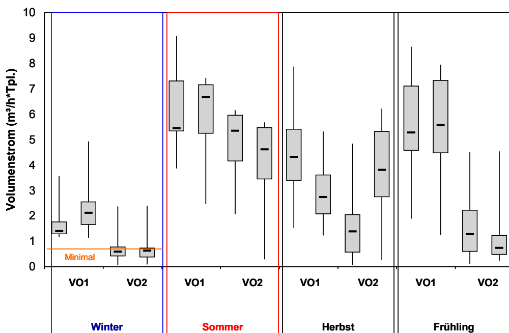
Abbildung 19: Mittelwert (Median), 25 %- und 75 %-Quantil, Minimum sowie Maximum des stündlichen Volumenstromes je Tierplatz innerhalb des MZF zu den Klimafenstern Winter, Sommer, Herbst und Frühling in den Volierehaltungen
