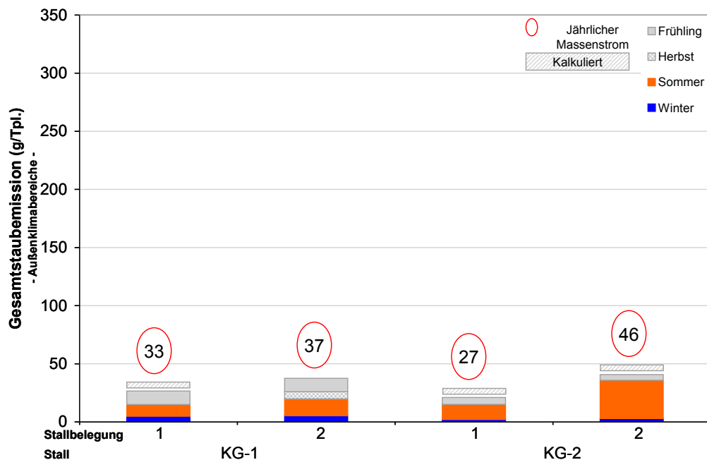
Abbildung 14: Berechneter Gesamtstaubmassenstrom je Tierplatz innerhalb der Klimafenster Winter, Sommer, Herbst und Frühling sowie über ein Jahr für die Kleingruppenhaltungen
