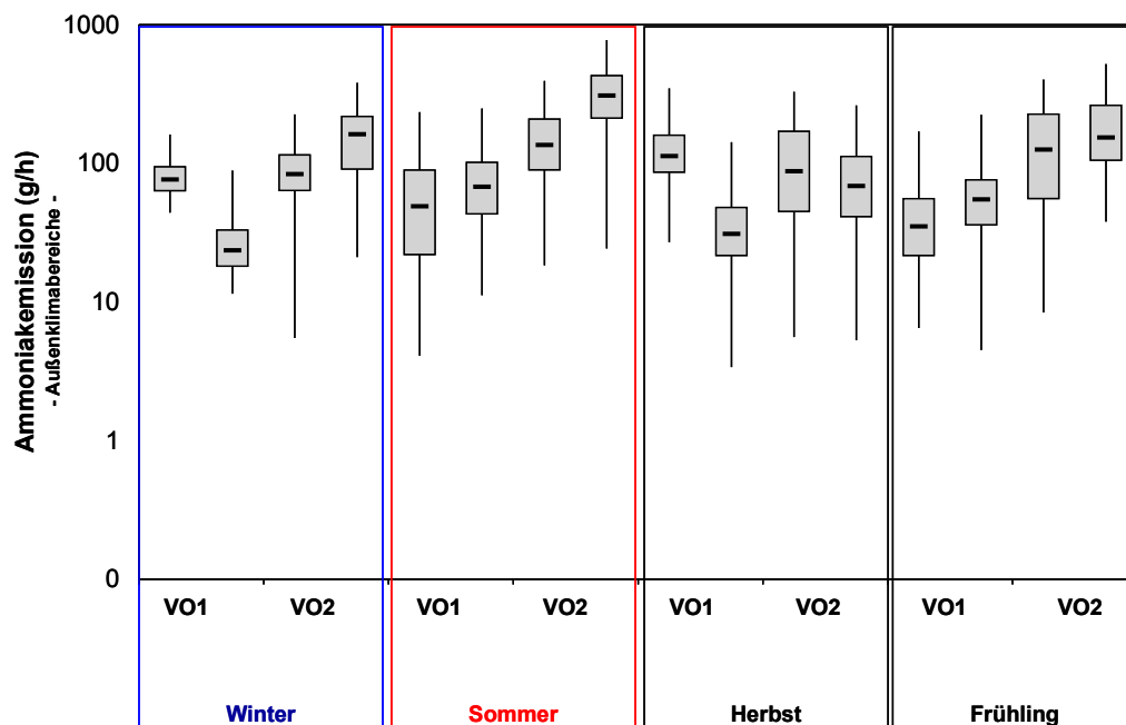
Abbildung 20: Mittelwert (Median), 25 %- und 75 %-Quantil, Minimum sowie Maximum des stündlichen Ammoniakmassenstromes innerhalb des MZF zu den Klimafenstern Winter, Sommer, Herbst und Frühling in den Volierehaltungen
