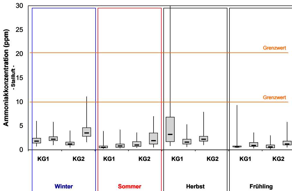
Abbildung 10: Mittelwert (Median), 25 %- und 75 %-Quantil, Minimum sowie Maximum der Ammoniakkonzentration in der Stallluft innerhalb des MZF zu den Klimafenstern Winter, Sommer, Herbst und Frühling in den Kleingruppenhaltungen
