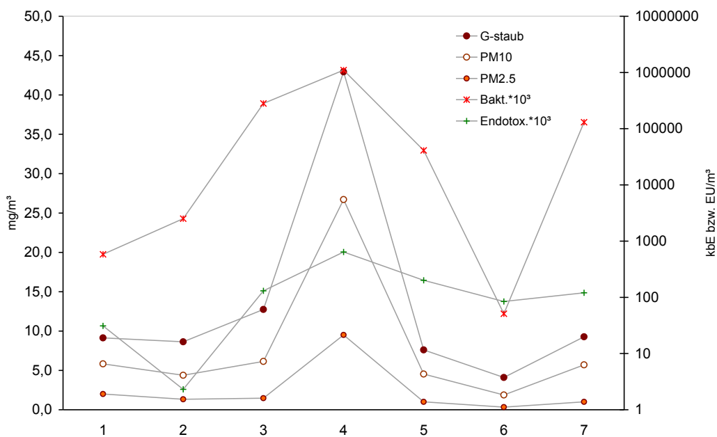
Abb. A-3: Zusammenhänge zwischen den Messwerten Gesamtstaub, Fraktionen PM10 sowie PM2,5 und den luftgetragenen Bakterien und Endotoxinen im Abluftstrom am Beispiel der VO-1 (<15.000 Tpl.)
