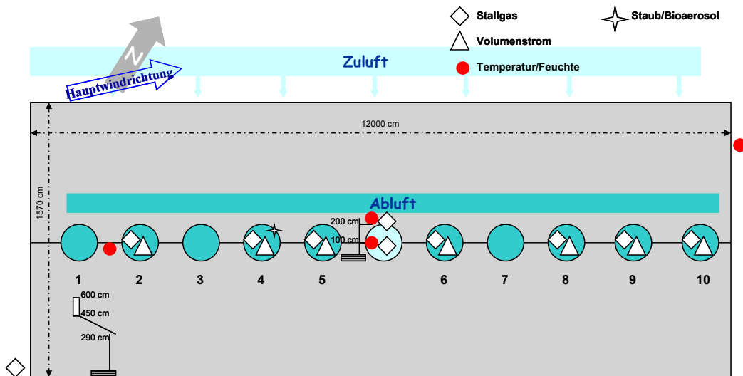
Abbildung 2: Messpunkteplan in der Bodenhaltung VO-2 (> 15.000 Tpl.)
