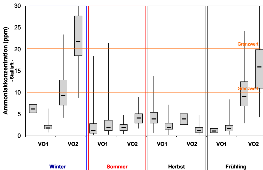
Abbildung 18: Mittelwert (Median), 25 %- und 75 %-Quantil, Minimum sowie Maximum der Ammoniakkonzentration in der Stallluft innerhalb des MZF zu den Klimafenstern Winter, Sommer, Herbst und Frühling in den Volierehaltungen
