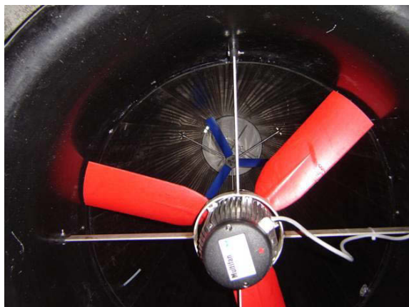
Abbildung 6: Abluftkamin mit Ventilator (rot) und Messventilator (blau)
