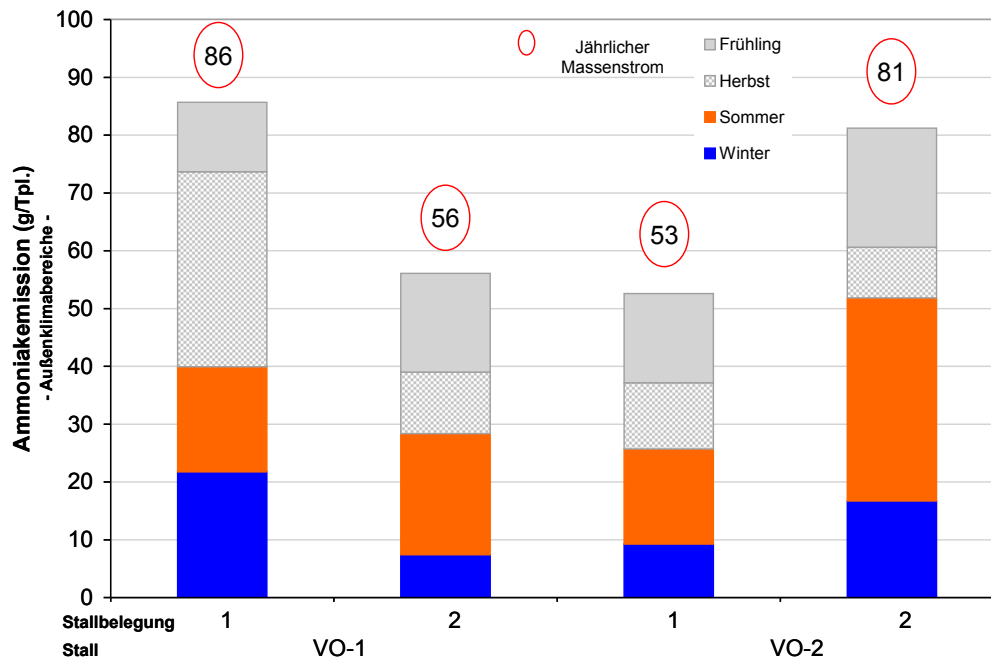
Abbildung 21: Berechneter Ammoniakmassenstrom je Tierplatz innerhalb der Klimafenster Winter, Sommer, Herbst und Frühling sowie über ein Jahr für die Volierehaltungen
