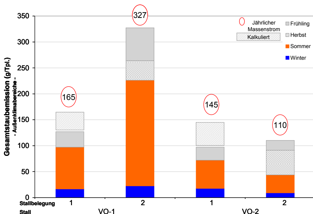
Abbildung 22: Berechneter Gesamtstaubmassenstrom je Tierplatz innerhalb der Klimabereiche Winter, Sommer, Herbst und Frühling sowie über ein Jahr für die Volierehaltungen
