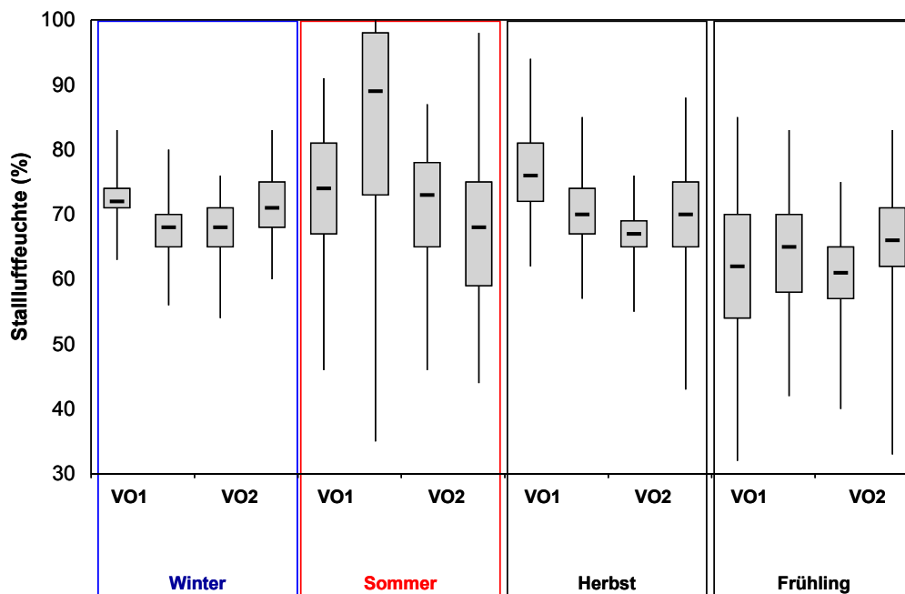
Abbildung 17: Mittelwert (Median), 25 %- und 75 %-Quantil, Minimum sowie Maximum der Stallluftfeuchte innerhalb des MZF zu den Klimafenstern Winter, Sommer, Herbst und Frühling in den Volierehaltungen
