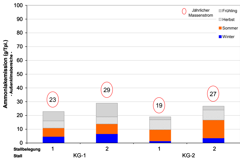
Abbildung 13: Berechneter Ammoniakmassenstrom je Tierplatz innerhalb der Klimafenster Winter, Sommer, Herbst und Frühling sowie über ein Jahr für die Kleingruppenhaltungen
