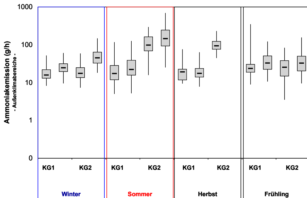
Abbildung 12: Mittelwert (Median), 25 %- und 75 %-Quantil, Minimum sowie Maximum des stündlichen Ammoniakmassenstromes innerhalb des MZF zu den Klimafenstern Winter, Sommer, Herbst und Frühling in den Kleingruppenhaltungen
