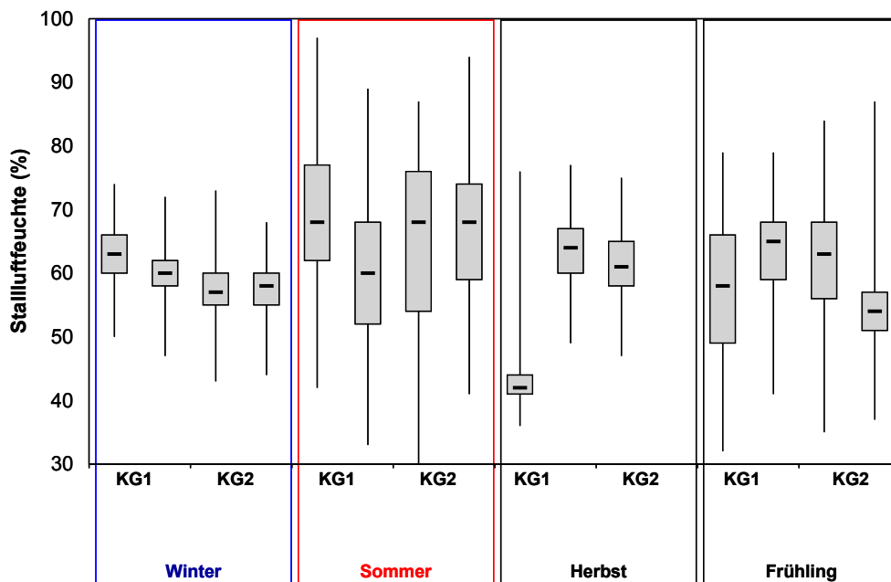
Abbildung 9: Mittelwert (Median), 25 %- und 75 %-Quantil, Minimum sowie Maximum der Stallluftfeuchte innerhalb des MZF zu den Klimafenstern Winter, Sommer, Herbst und Frühling in den Kleingruppenhaltungen
