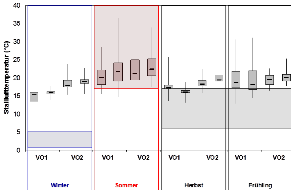
Abbildung 16: Mittelwert (Median), 25 %- und 75 %-Quantil, Minimum sowie Maximum der Stalllufttemperatur innerhalb des MZF zu den Klimafenstern Winter, Sommer, Herbst und Frühling in den Volierehaltungen
