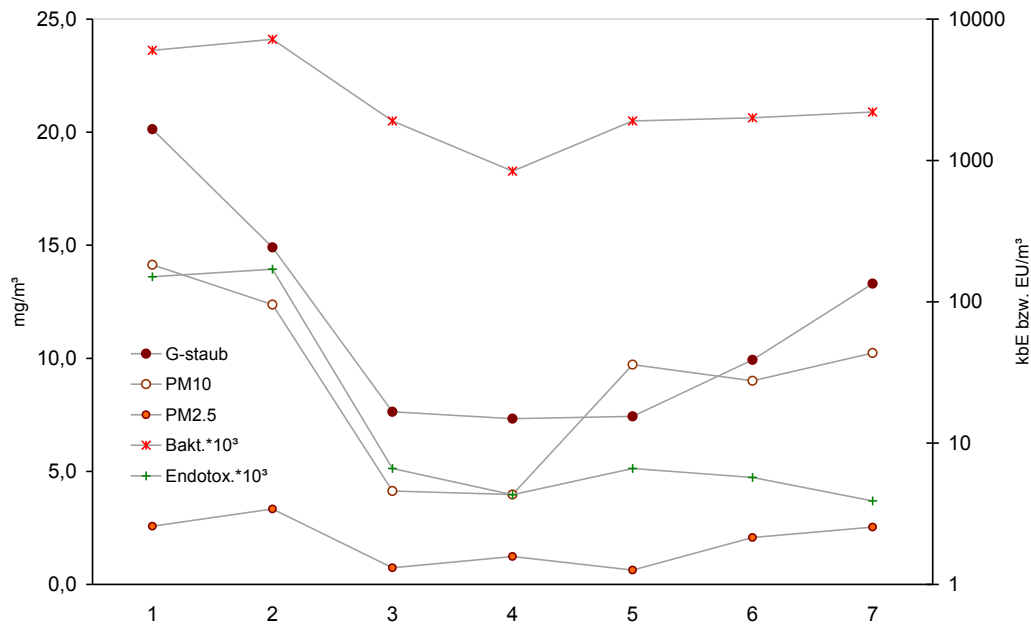
Abbildung 15: Zusammenhänge zwischen den Messwerten Gesamtstaub, Fraktionen PM10 sowie PM2,5 und den luftgetragenen Bakterien und Endotoxinen im Abluftstrom am Beispiel der VO-2 (>15.000 Tpl.)
