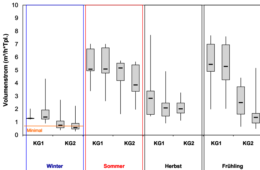
Abbildung 11: Mittelwert (Median), 25 %- und 75 %-Quantil, Minimum sowie Maximum des stündlichen Volumenstromes je Tierplatz innerhalb des MZF zu den Klimafenstern Winter, Sommer, Herbst und Frühling in den Kleingruppenhaltungen
