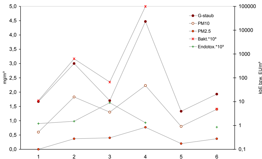
Abb. A-1: Zusammenhänge zwischen den Messwerten Gesamtstaub, Fraktionen PM10 sowie PM2,5 und den luftgetragenen Bakterien und Endotoxinen im Abluftstrom am Beispiel der KG-2 (>15.000 Tpl.)
