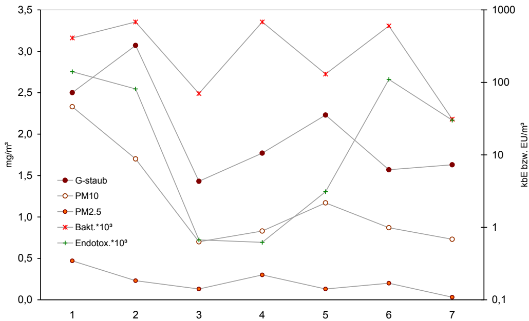
Abb. A-2: Zusammenhänge zwischen den Messwerten Gesamtstaub, Fraktionen PM10 sowie PM2,5 und den luftgetragenen Bakterien und Endotoxinen im Abluftstrom am Beispiel der KG-1 (<15.000 Tpl.)
