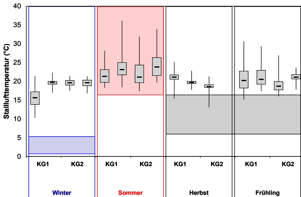
Abbildung 8: Mittelwert (Median), 25 %- und 75 %-Quantil, Minimum sowie Maximum der Stalllufttemperatur innerhalb des MZF zu den Klimafenstern Winter, Sommer, Herbst und Frühling in den Kleingruppenhaltungen
