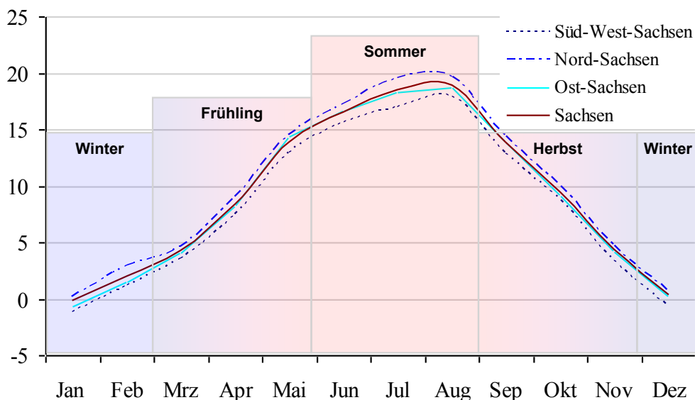
Abbildung 1: Langjährig gemessene mittlere Lufttemperatur in Sachsen im Jahresverlauf
