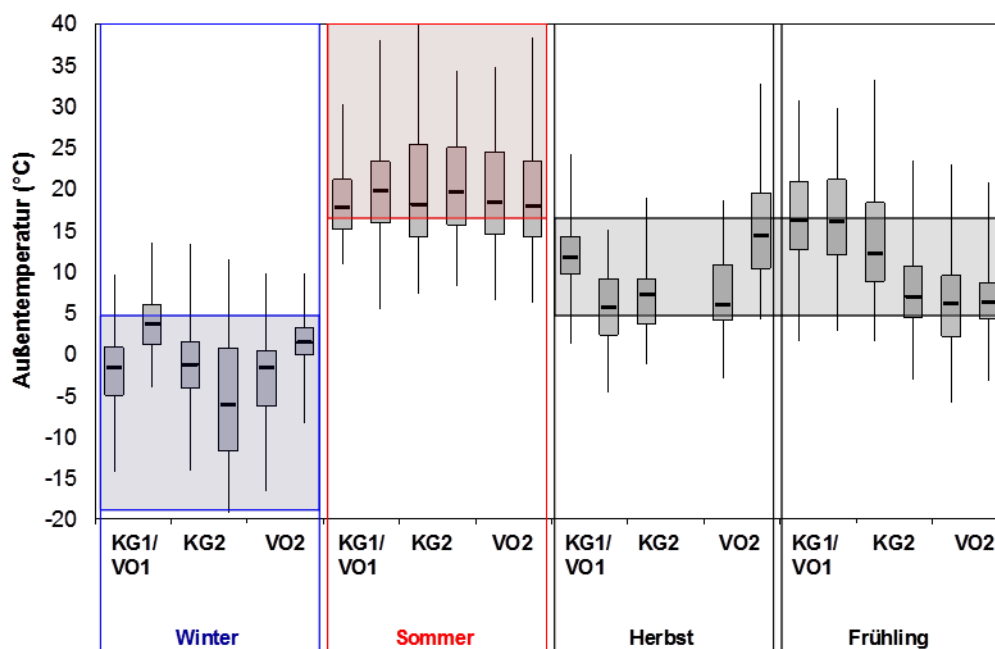
Abbildung 5: Quartile sowie Minimum und Maximum der Außenlufttemperatur innerhalb der Messzeitfenster für die Klimafenster
