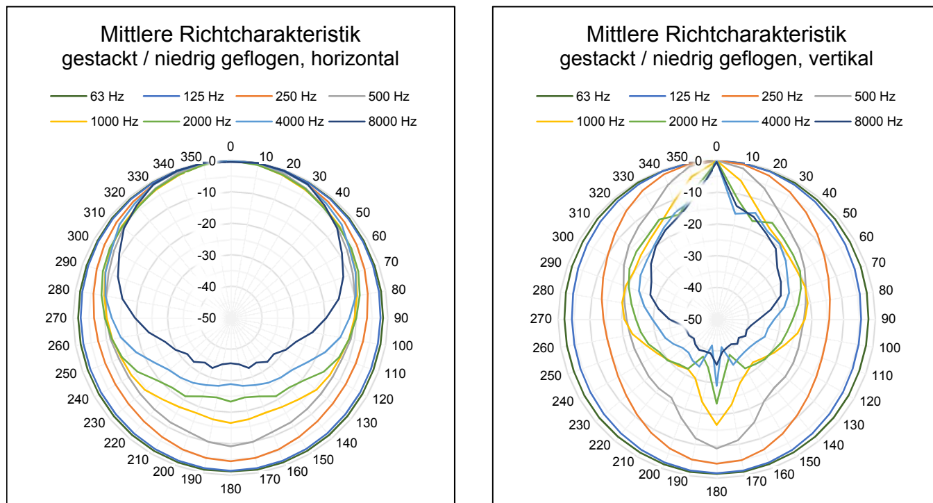
Abbildung 3: Simulierte mittlere horizontale und vertikale Richtcharakteristik von gestackten bzw. niedrig geflogenen Line Arrays, oktawweise
