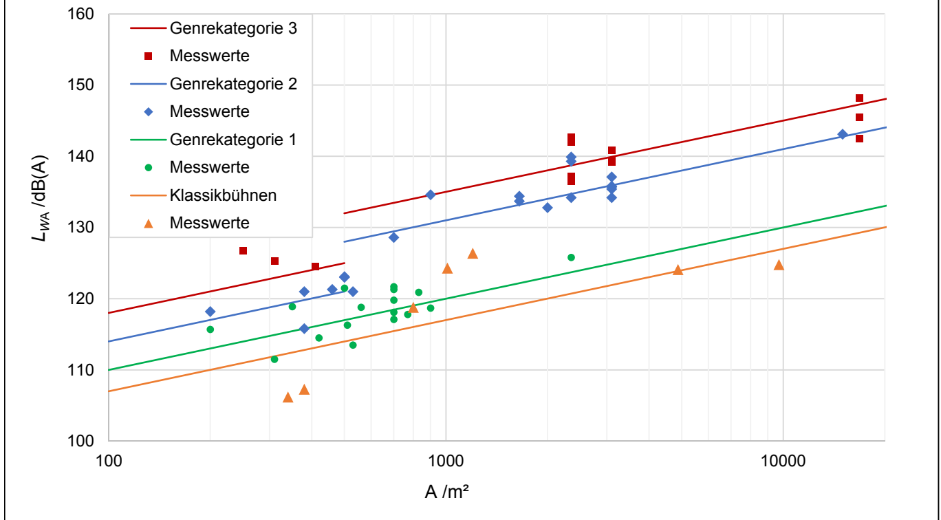
Abbildung 12: Prognosegeraden für den Schalleistungspegel der drei untersuchten Genrekategorien auf Klein- und Großbühnen sowie der untersuchten Klassikbühnen im Vergleich zu aus Messungen ermittelten Werten
