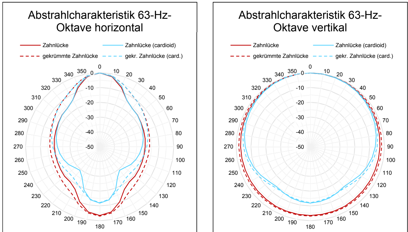
Abbildung 21: Simulierte horizontale und vertikale Richtcharakteristik für die 63-Hz-Oktave von acht doppelt gestackten Subwooferclustern in Zahnlückenordnung (gerade/gekrümmt)
