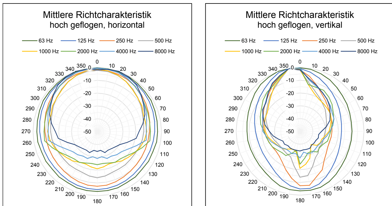
Abbildung 4: Simulierte mittlere horizontale und vertikale Richtcharakteristik von hoch geflogenen Line Arrays, oktawweise
