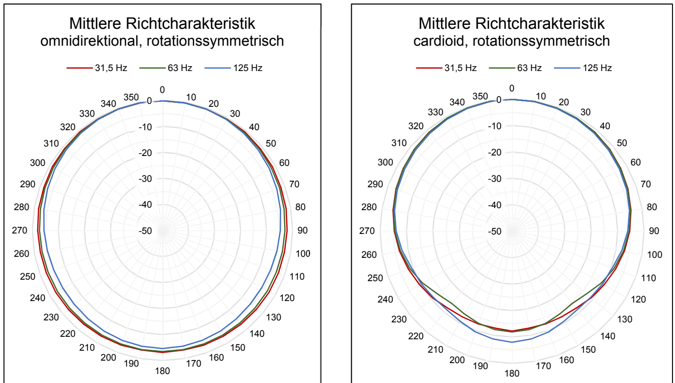
Abbildung 7: Simulierte mittlere, rotationssymmetrische Richtcharakteristik von omnidirektionalen und Cardioid-Subwoofern, oktavweise
