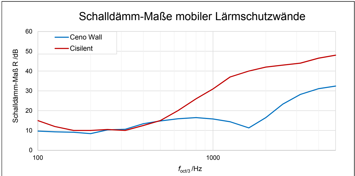
Abbildung 27: Schalldämm-Maße zweier mobiler Lärmschutzwände
