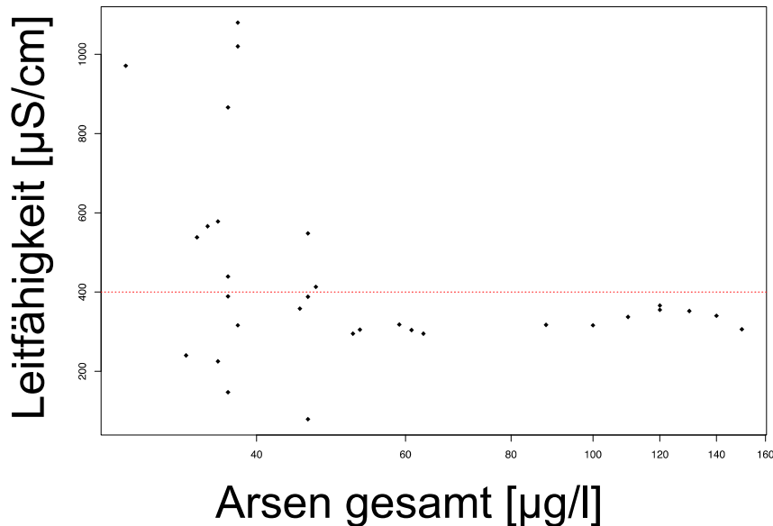
Abbildung 27: Arsen gesamt und elektrische Leitfähigkeit, LAWA-Typ 5, sächsische Daten, Werte oberhalb des 98-Perzentils von Arsen gesamt , N = 31; rot gepunktete Linie = oberer Leitfähigkeitsschwellenwert des Gewässertyps
