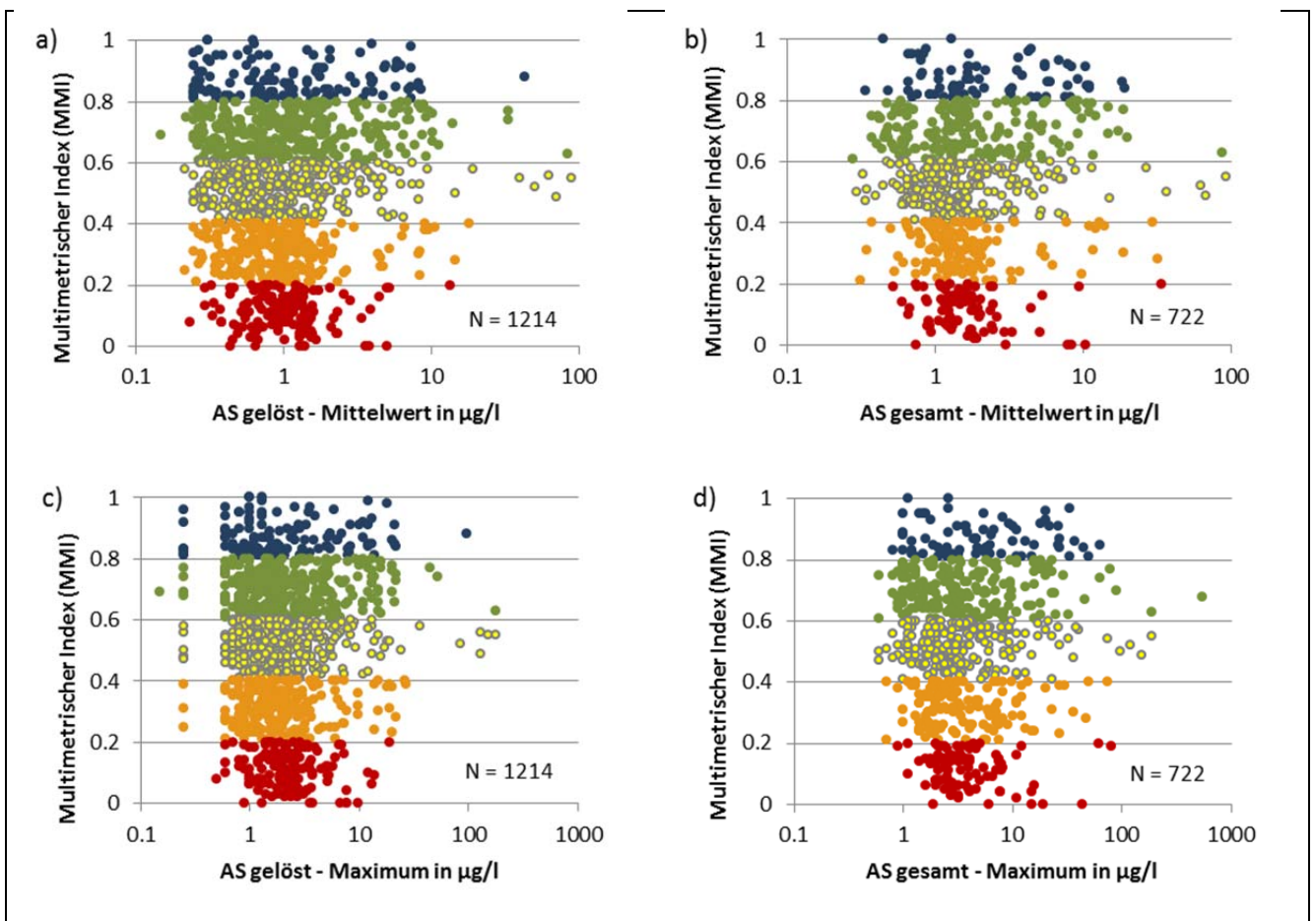
Abbildung 35: Multimetriche Index in Abhängigkeit der Arsenkonzentration. Die jeweiligen Zustandsklassen sind nach dem offiziellen Farbcode entsprechend gekennzeichnet.
