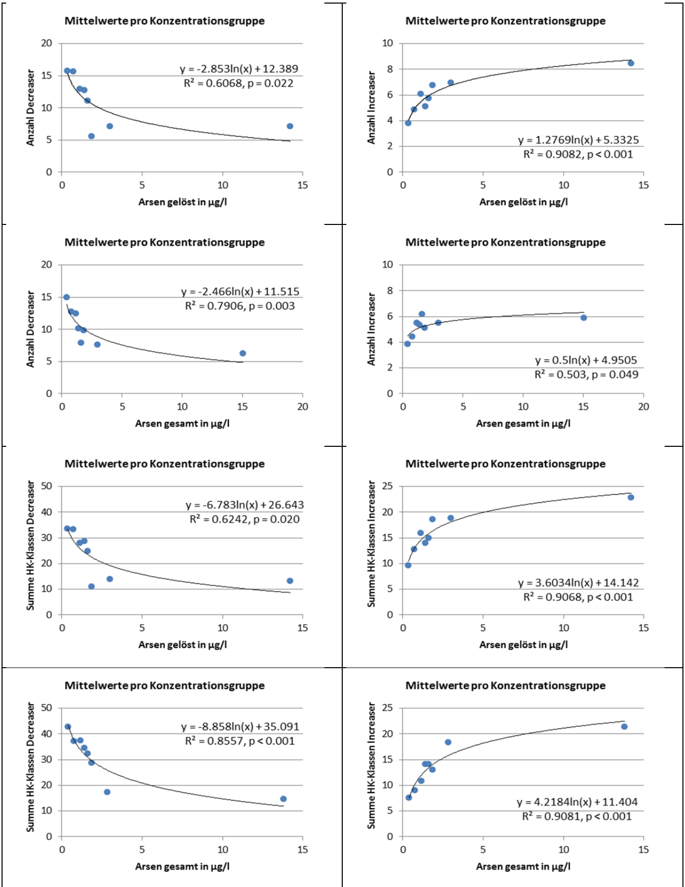
Abbildung 102: Abgeleitete Funktionen für Makrozoobenthos.
