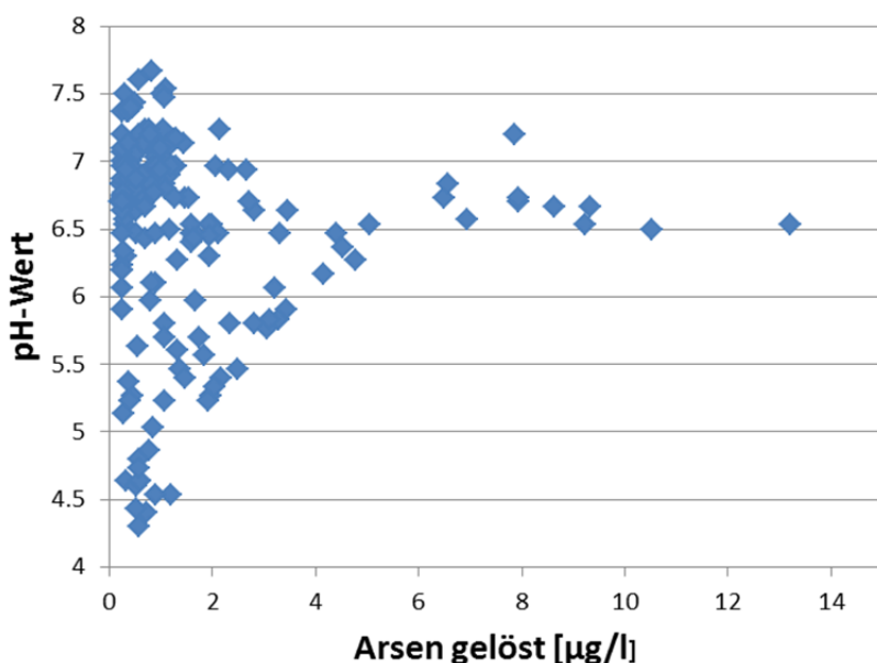
Abbildung 91: pH-Wert in Abhängigkeit der gelösten Arsenkonzentration, gezeigt für ACP-Referenzgewässer.
