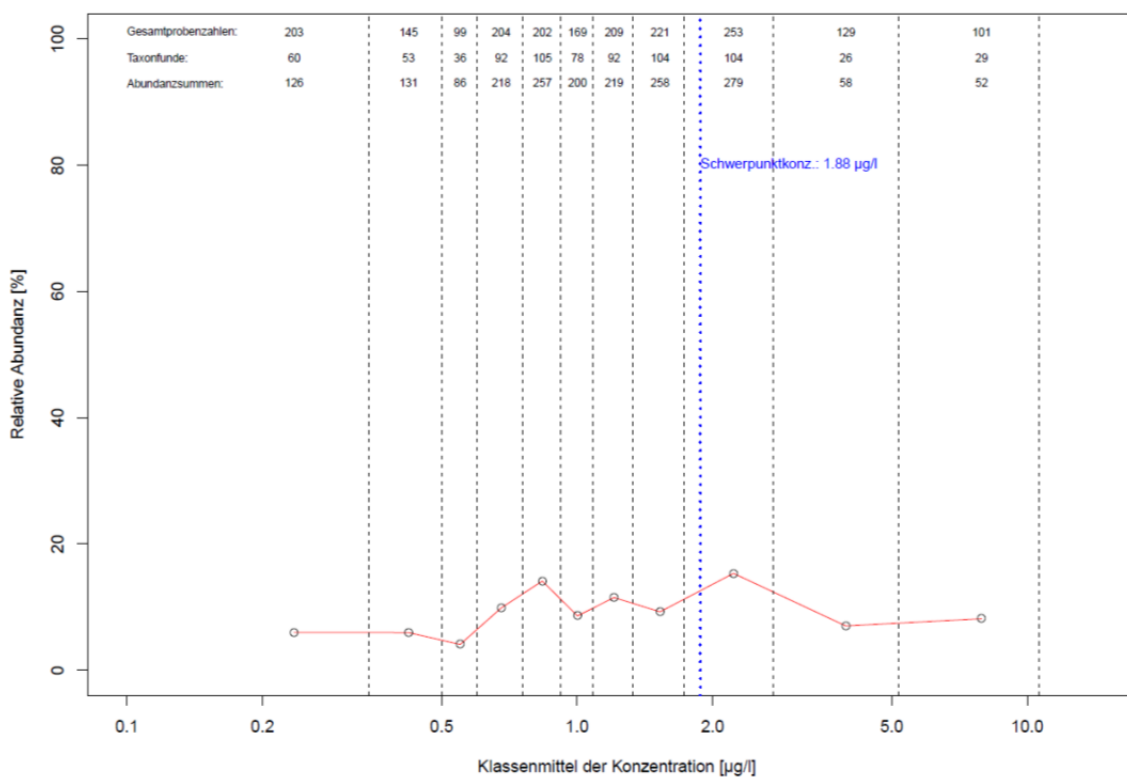
Abbildung 44: Gemittelte relative Abundanz des Taxon Asellus aquaticus in Abhängigkeit von Arsen gesamt
