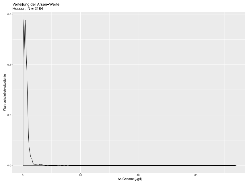
Abbildung 7: Wahrscheinlichkeitsdichtefunktion der Arsengehalte in Fließgewässern Hessens (Datengrundlage: HLNUG)
