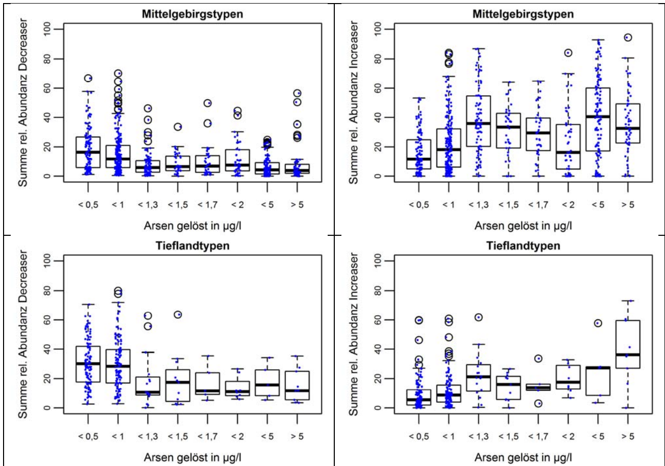
Abbildung 101: Summe der relativen Abundanz der De- und Inreaser der Diatomeen in unterschiedlichen Fließgewässertypengruppen in Abhängigkeit der gemessenen Arsenkonzentration.
