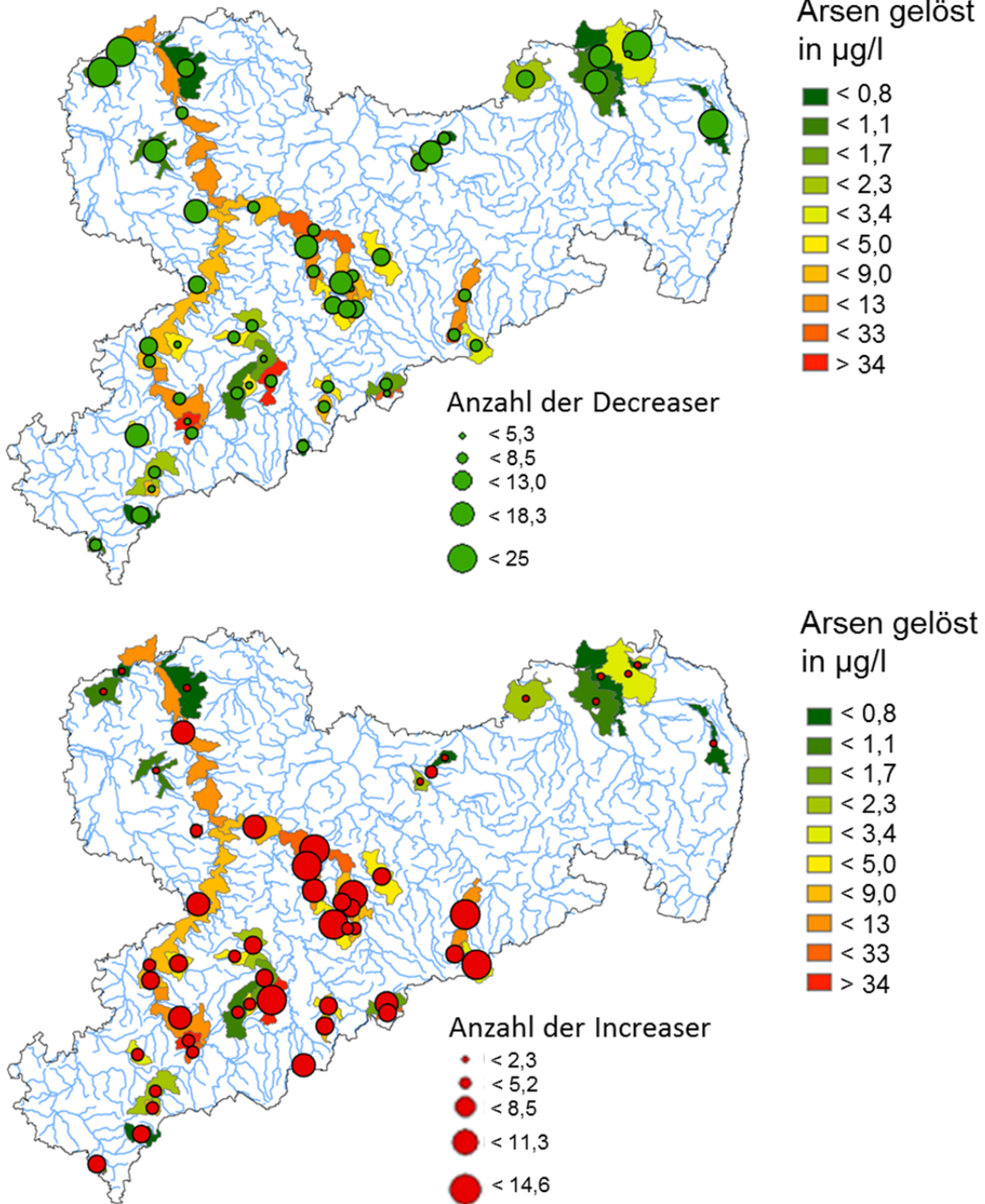
Abbildung 107: Mittlere Anzahl der De- und Increaser des Makrozoobenthos in den OWK der Gebietskulisse
