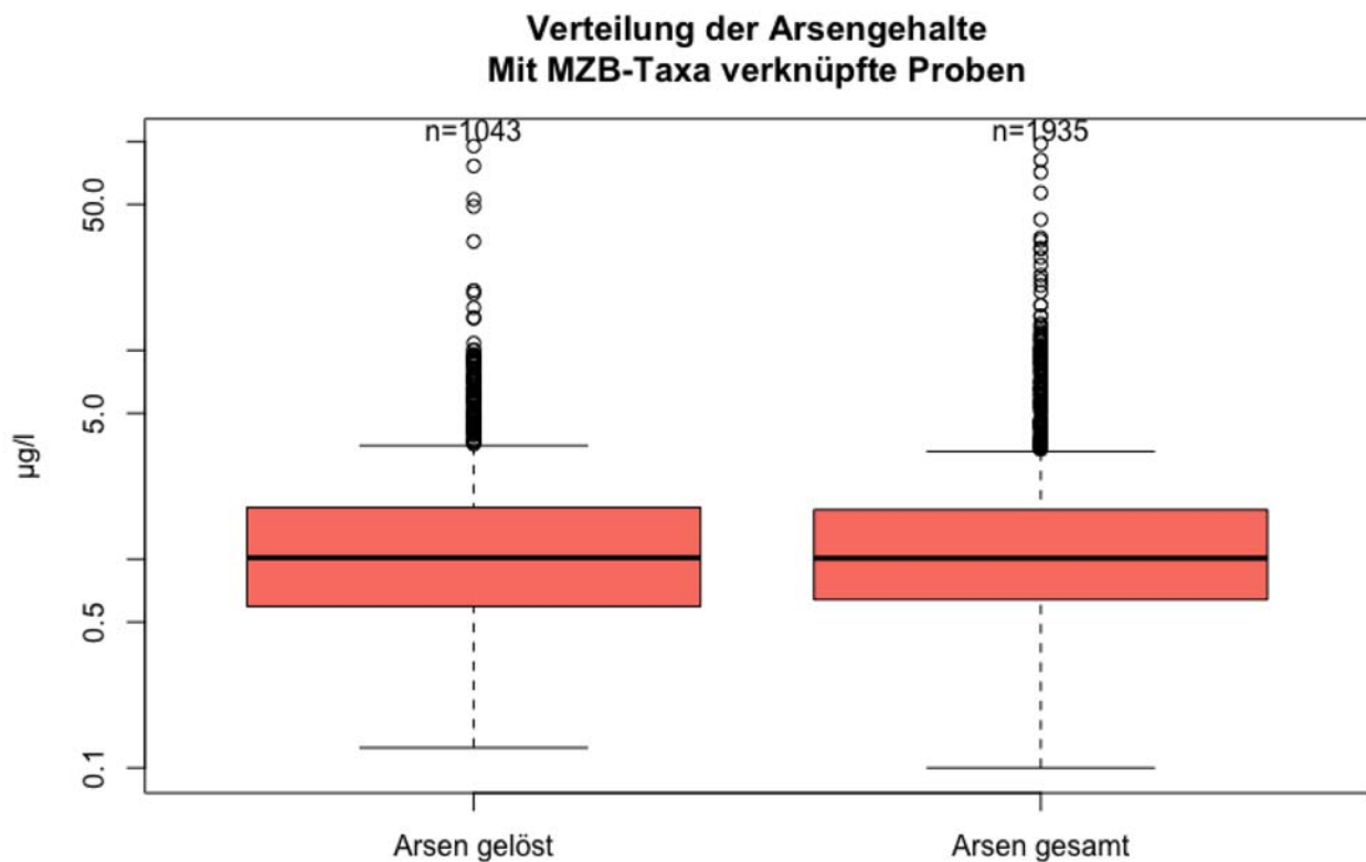
Abbildung 24: Verteilung der Arsengehalte der nur mit MZB-Taxafunden verknüpften aber nicht bewerteten Proben
