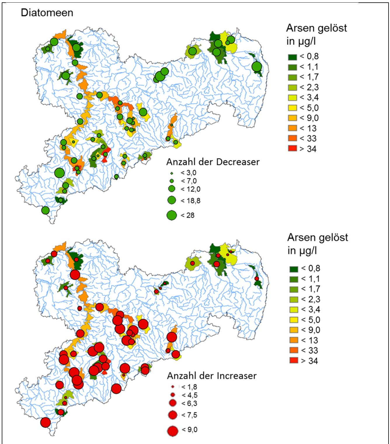
Abbildung 108: Mittlere Anzahl der De- und Increaser der Diatomeen in den OWK der Gebietskulisse
