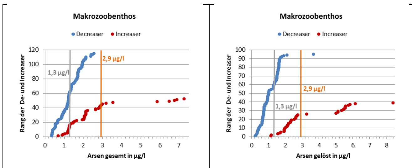
Abbildung 90: Schwellenwerte der Makrozoobenthos-Taxa für Arsen gesamt und Arsen gelöst , berechnet für die mittlere Arsenkonzentration. Jeder blaue Punkt entspricht dem Schwellenwert eines Decreasers, jeder rote Punkt dem Schwellenwert eines Increasers. Die Schwellenwerte der De- und Increaser sind in aufsteigender Reihenfolge (nach Rang) sortiert. Der Vorschlagswert der JD-UQN fw für Deutschland von 1,3 µg/l und die in von der Bundesregierung am 16.12.2015 beschlossene Fassung der OGewV enthaltene JD-UQN fw von 2,9 µg/l sind als vertikale Linien in grau und orange dargestellt.
