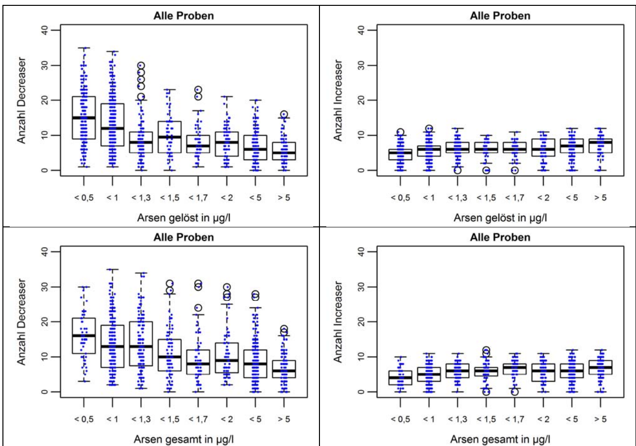
Abbildung 99: Anzahl der De- und Increaser der Diatomeen in Abhängigkeit der gemessenen Arsenkonzentration.
