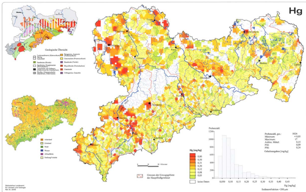
Abb. 4.1.8-2: Quecksilber in Bachsedimenten Sachsens
