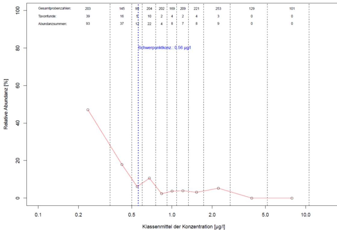
Abbildung 58: Gemittelte relative Abundanz des Taxon Baetis niger in Abhängigkeit von Arsen gesamt
