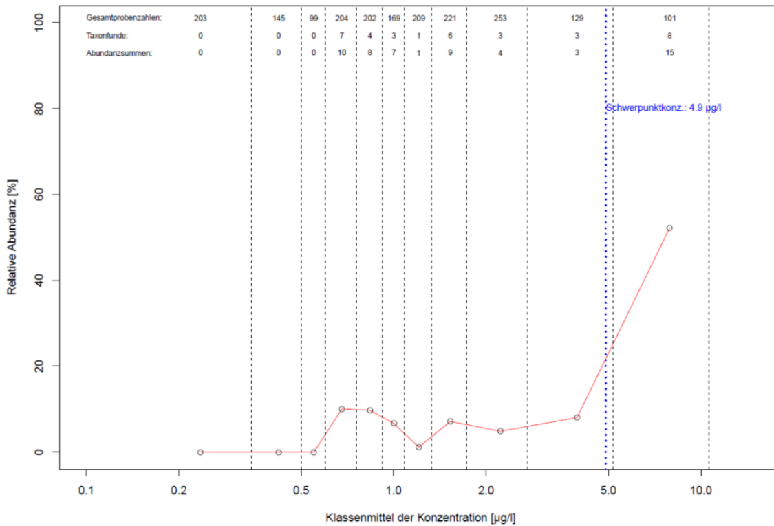
Abbildung 67: Gemittelte relative Abundanz des Taxon Oecetis notata in Abhängigkeit von Arsen gesamt
