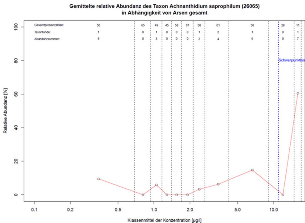
Abbildung 88: Gemittelte relative Abundanz des Taxon Achnanthydium saprophilum in Abhängigkeit von Arsen gesamt
