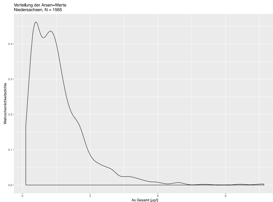
Abbildung 8: Wahrscheinlichkeitsdichtefunktion der Arsengehalte in Fließgewässern Niedersachsens (Datengrundlage: NLWKN)
