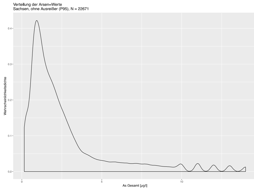
Abbildung 11: Wahrscheinlichkeitsdichtefunktion der Arsengehalte in Fließgewässern Sachsens, unteres 95-Perzentil (Datengrundlage: LfULG)
