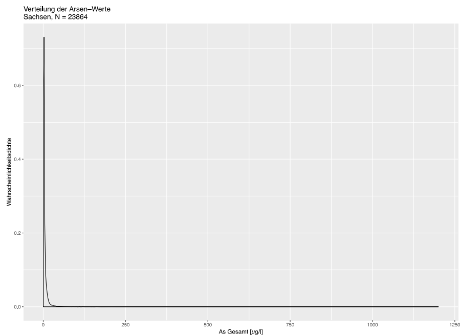
Abbildung 10: Wahrscheinlichkeitsdichtefunktion der Arsengehalte in Fließgewässern Sachsens (Datengrundlage: LfULG)
