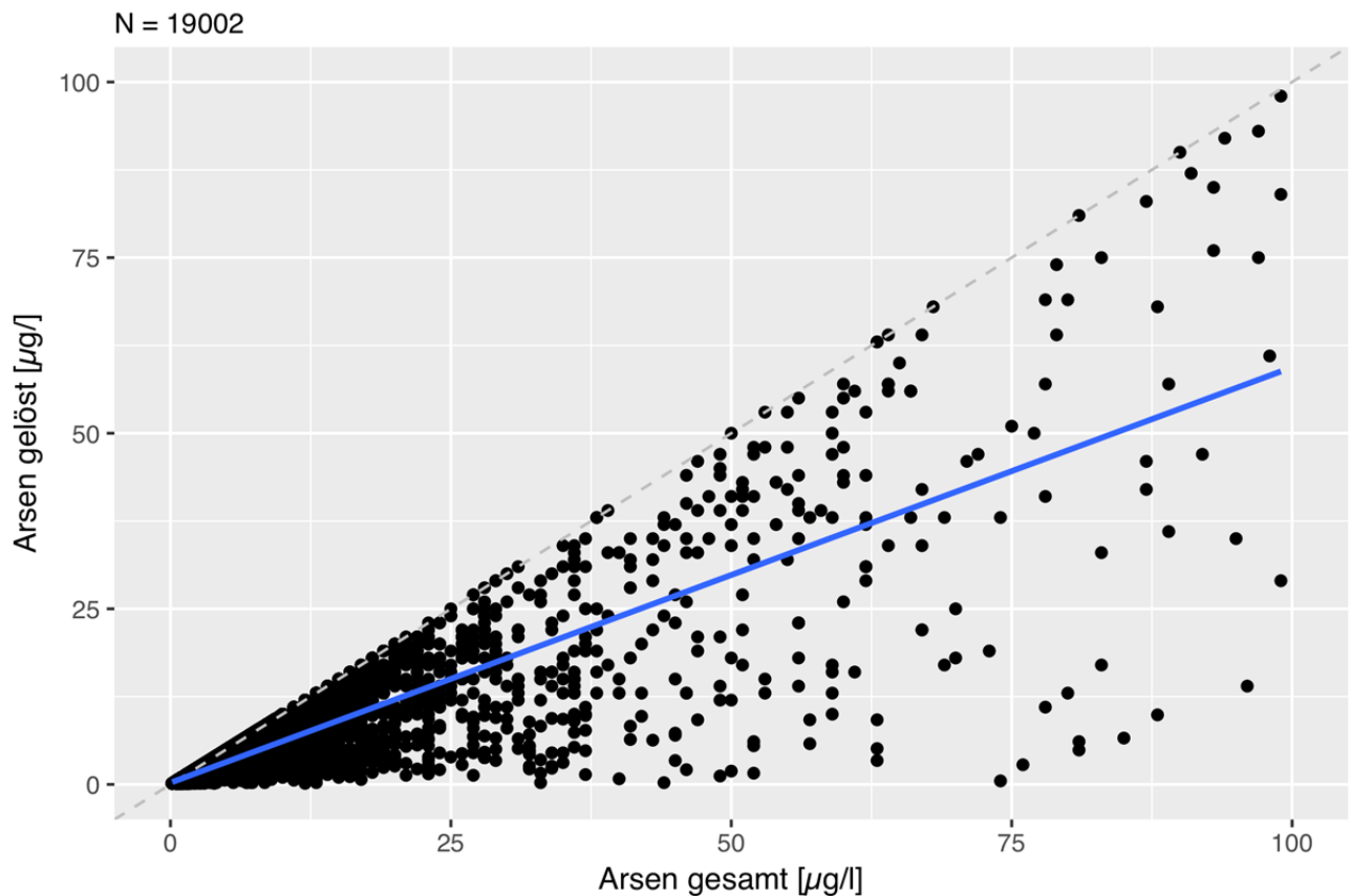
Abbildung 31: Streudiagramm Arsen gelöst zu Arsen gesamt (Detailansicht: Konzentration < 100 µg/l, Datengrundlage: LfULG, 2016)
