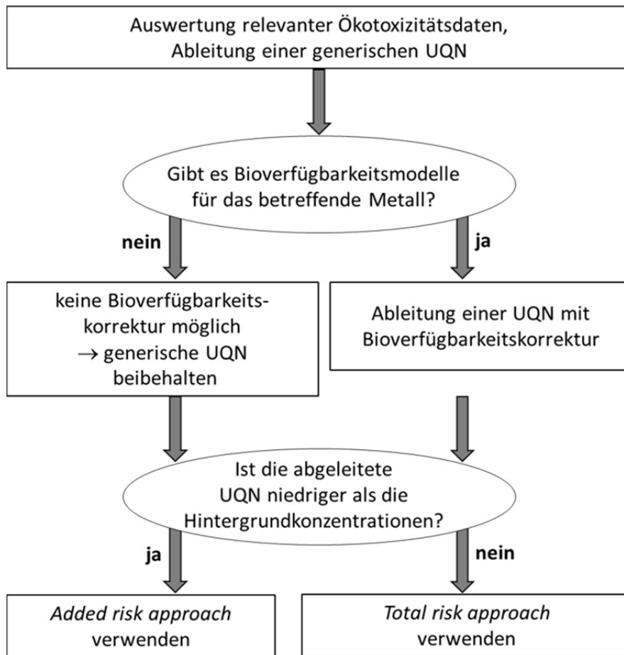
Abbildung 18: Übersicht über die grundlegende Vorgehensweise bei der Ableitung von Umweltqualitätsnormen (UQN) für Metalle (basierend auf EC 2011, vereinfacht). Zusätzliche Informationen zur Vorgehensweise: siehe Text.
