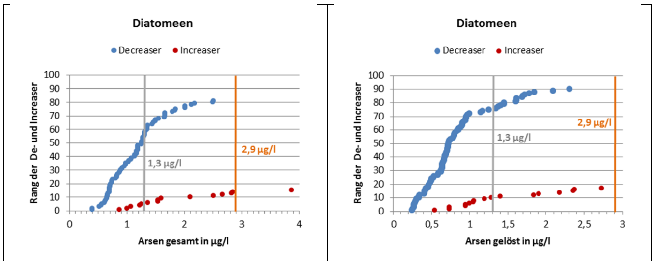
Abbildung 92: Schwellenwerte der Diatomeen-Taxa für Arsen gesamt und Arsen gelöst , berechnet für die mittlere Arsenkonzentration. Jeder blaue Punkt entspricht dem Schwellenwert eines Decreasers, jeder rote Punkt dem Schwellenwert eines Increasers. Die Schwellenwerte der De- und Increaser sind in aufsteigender Reihenfolge (nach Rang) sortiert. Der Vorschlagswert der JD-UQN fw für Deutschland von 1,3 µg/l und die in von der Bundesregierung am 16.12.2015 beschlossene Fassung der OGewV enthaltene JD-UQN fw von 2,9 µg/l sind als vertikale Linien in grau und orange dargestellt.
