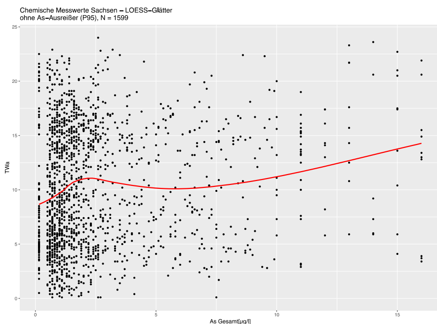
Abbildung 16: Streudiagramm Arsen und Wassertemperatur (ohne As-Ausreißer, Datengrundlage: LfULG, 2016)
