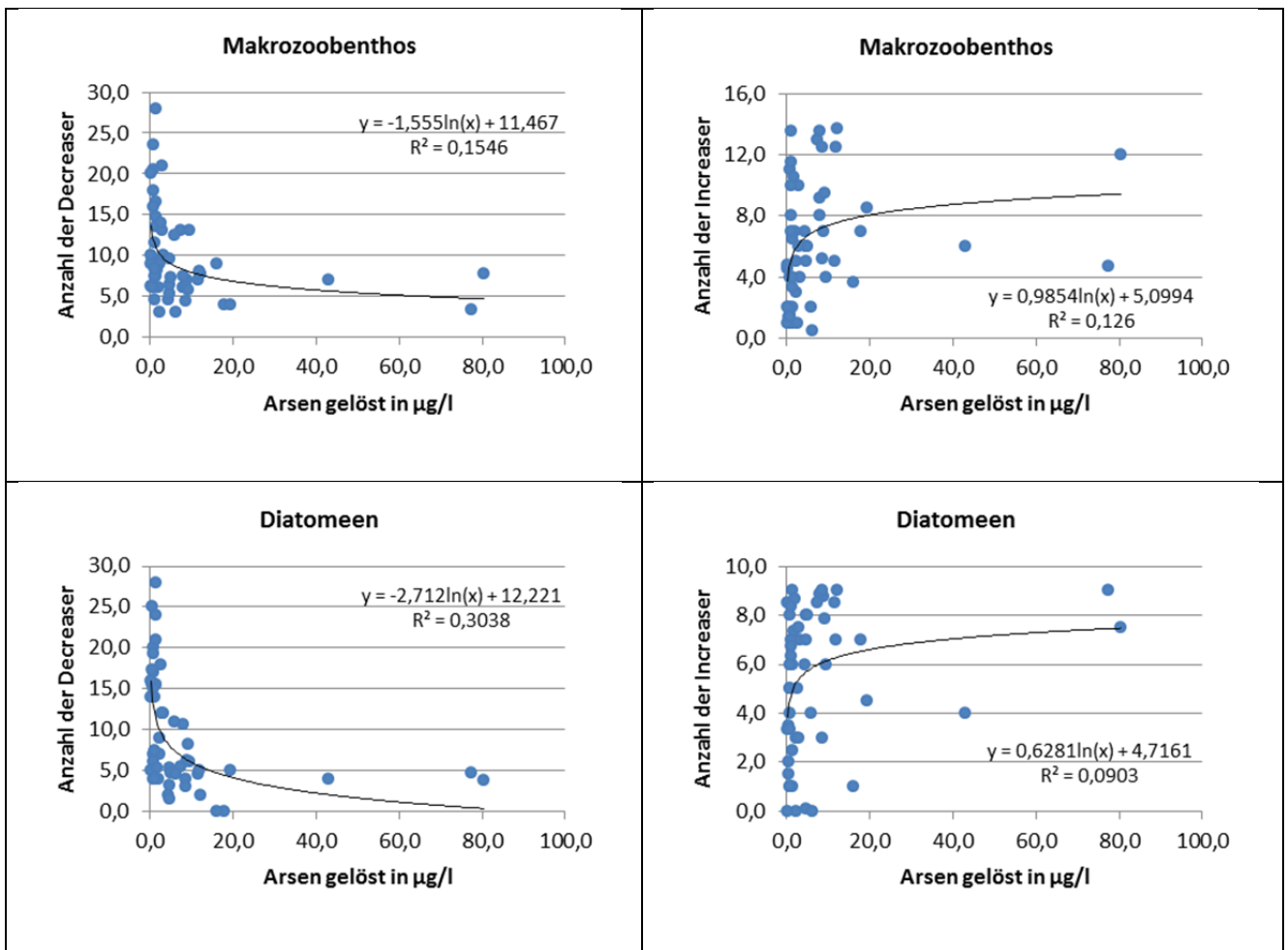
Abbildung 106: Anzahl der De- und Increaser in Proben der Gebietskulisse in Abhängigkeit der Arsenkonzentration
