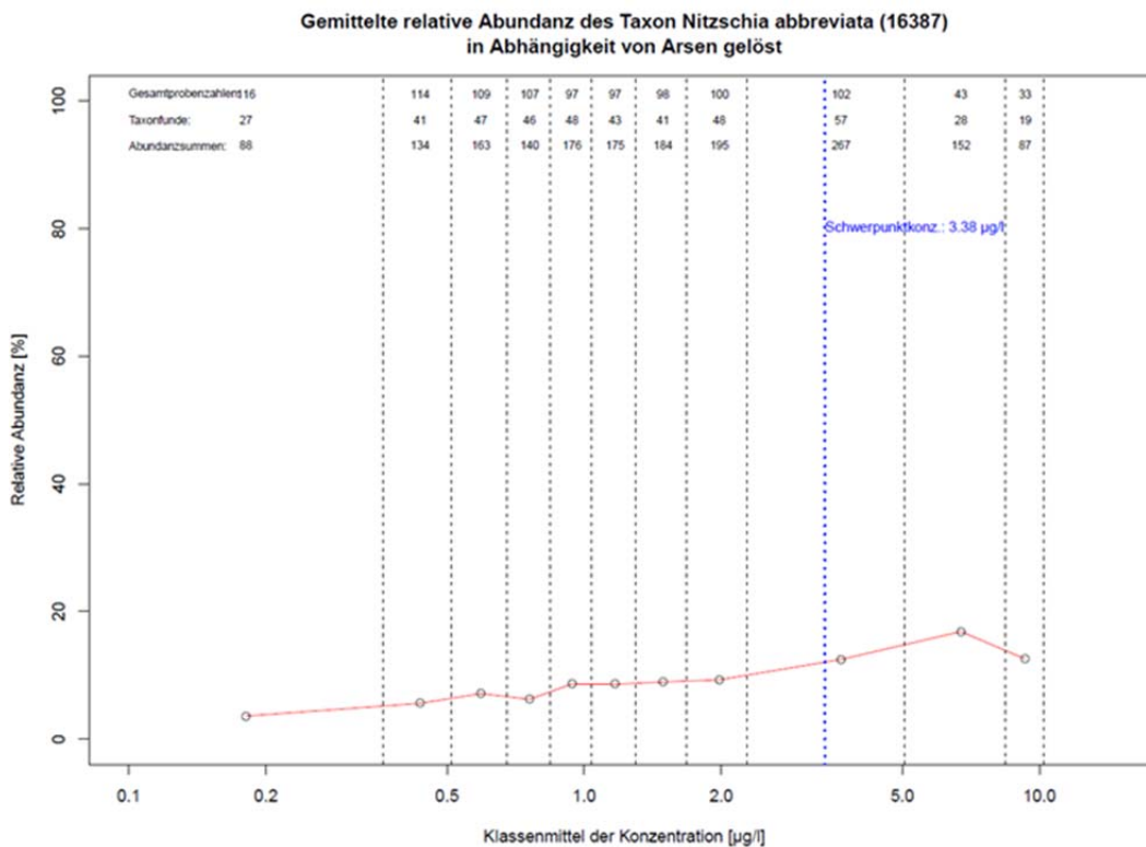
Abbildung 81: Gemittelte relative Abundanz des Taxon Nitzschia abbreviata in Abhängigkeit von Arsen gelöst
