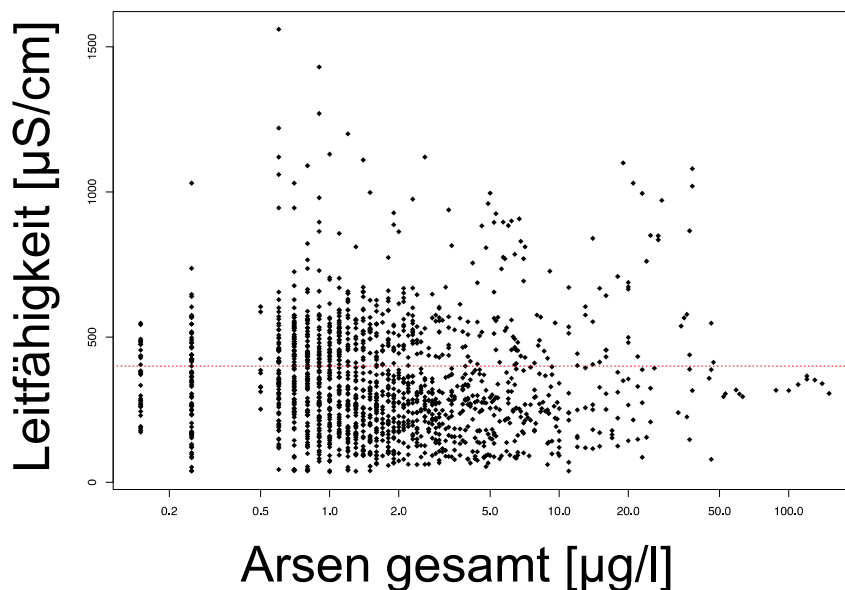
Abbildung 26: Arsen gesamt und elektrische Leitfähigkeit, LAWA-Typ 5, sächsische Daten, N = 1.538; rot gepunktete Linie = oberer Leitfähigkeitsschwellenwert des Gewässertyps
