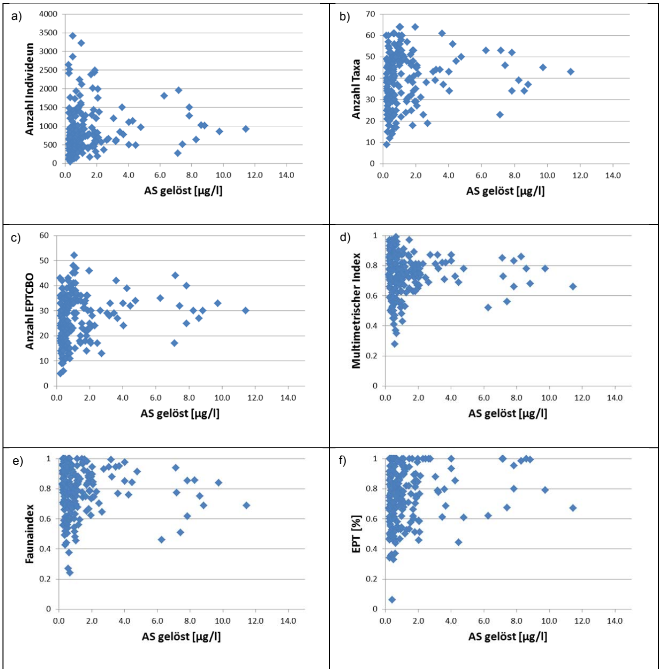
Abbildung 104: Ausgewählte Metrics (biozönotisch Kenngrößen) der Qualitätskomponente Makrozoobenthos in Abhängigkeit der Arsenkonzentration (Arsen gelöst ).
