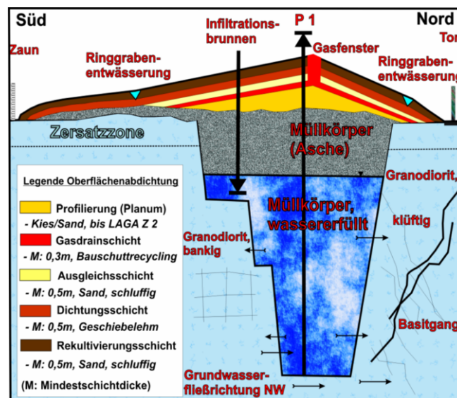
Abbildung 2: Anlagentechnik und mineralische Oberflächenabdeckung
