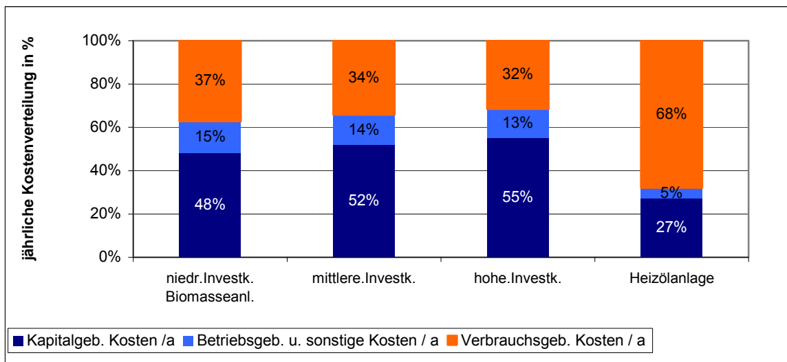
Abbildung 83: Kostenverteilung der jährlichen Gesamtkosten einer Holzhackschnitzelheizung bei unterschiedlicher Investitionskostenhöhe im Vergleich zu einer Heizölanlage/Kalthaus 2 500 m 2
