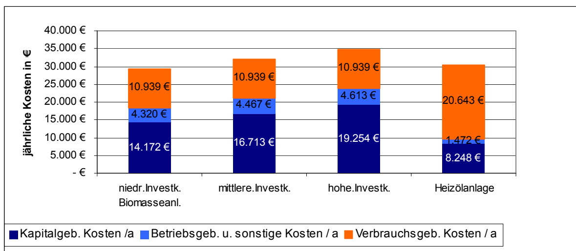
Abbildung 82: Jährliche Gesamtkosten einer Holzhackschnitzelheizung bei unterschiedlicher Investitionskostenhöhe im Vergleich zu einer Heizölanlage/Kalthaus 2 500 m 2
