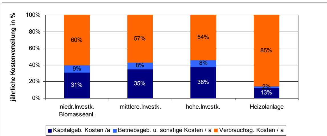
Abbildung 89: Kostenverteilung der jährlichen Gesamtkosten einer Holzackschnitzelheizung bei unterschiedlicher Investitionskostenhöhe im Vergleich zu einer Heizölanlage/Kalthaus 2 500 m 2
