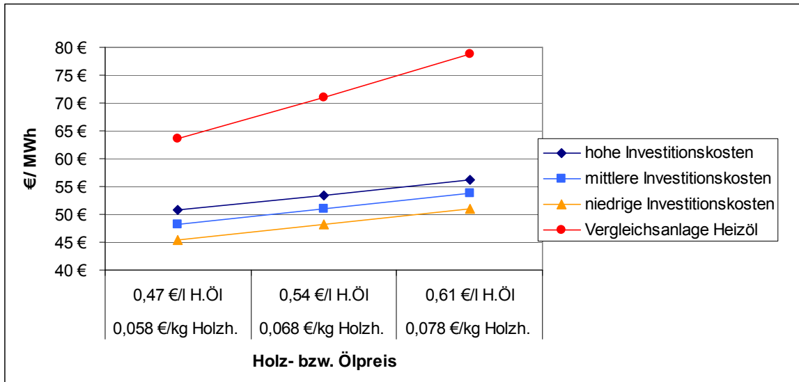
Abbildung 88: Wärmegestehungskosten in Euro/MWh für eine Holzackschnitzelanlage im Vergleich zu einer Heizölanlage bei verschiedenen Rahmenbedingungen/Warmhaus 2 500 m 2
