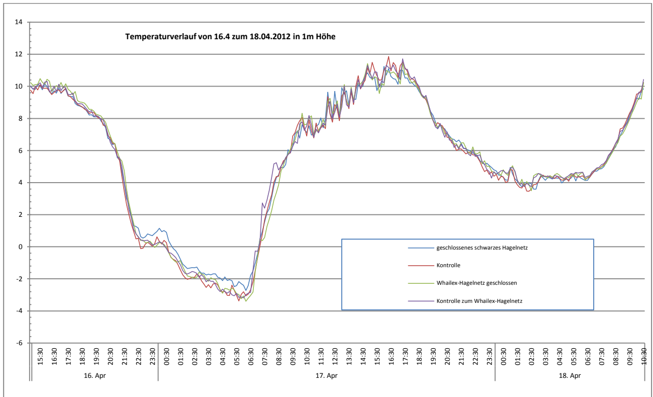
Abbildung 31: Temperaturverlauf 16. bis 18.04.2012
