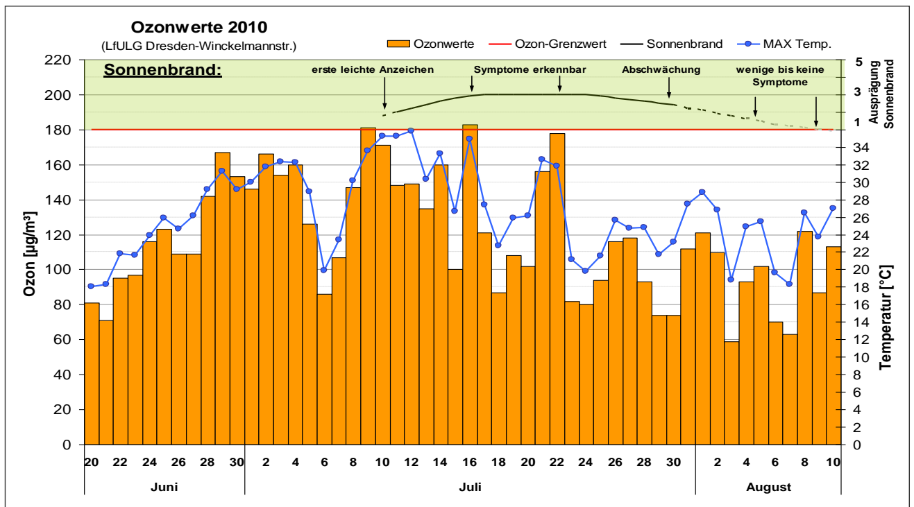
Abbildung 54: Ozongehalt und Temperatur im Sommer 2010
