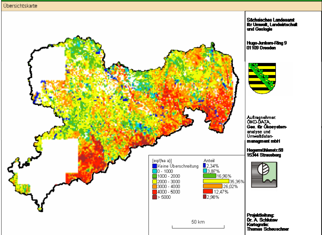
Abbildung 4: Überschreitung der Kritischen Belastungsgrenzen durch Säureeinträge im Jahr 2006
