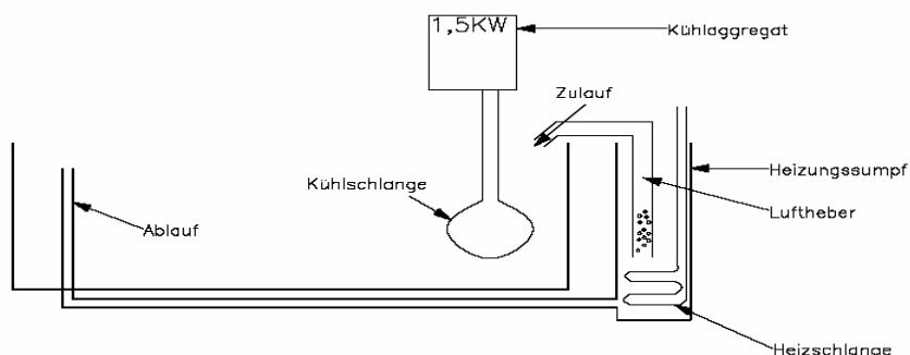
Abbildung 4: Schematische Darstellung des Kühlkreislaufs
