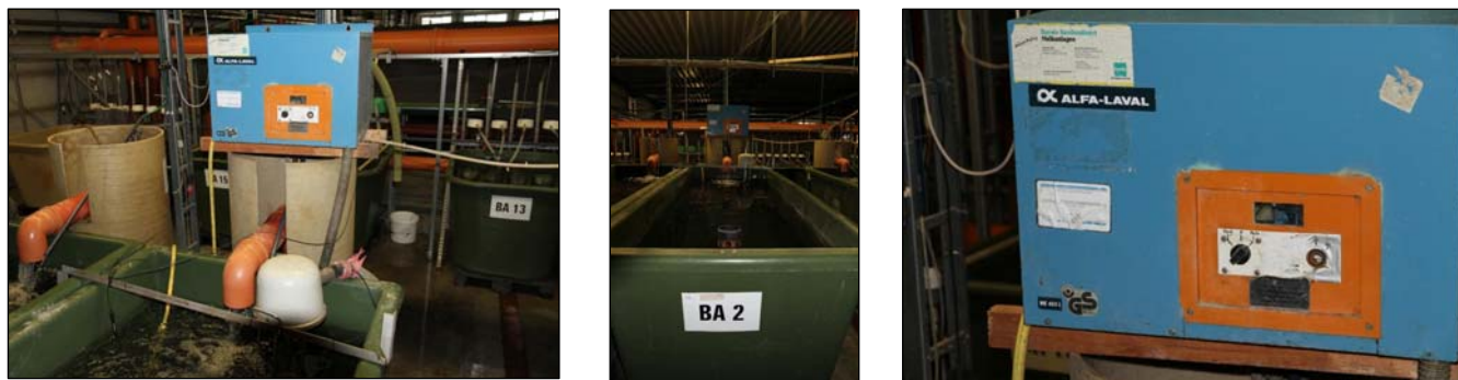
Abbildung 2: Kühlgerät ALFA LAVAL MK 403L (Leistung 1,5 KW) in den BA-Becken mit HSB-F1
