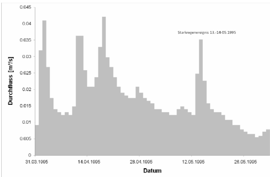
Abbildung 37: Abflussganglinie Hölzelbergbach 31.03.-30.04.1995
