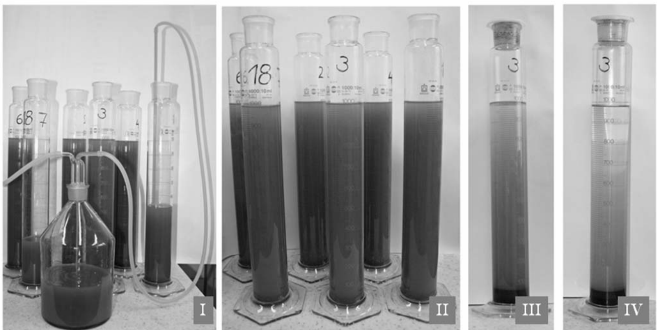
Abbildung 8: Durchführung des modifizierten Atterberg-Verfahrens
