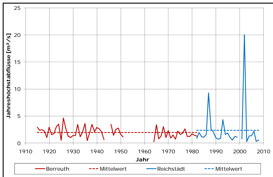
Abbildung 6: Jahreshöchstabflüsse der Pegel Reichstädt (PKZ 55152.1) und Berreuth (PKZ 55152.0) am Reichstädter Bach
