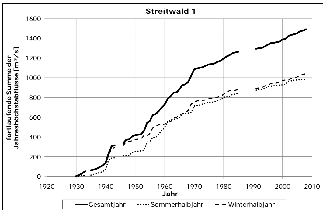
Abbildung 14: Summenlinien für den Pegel Streitwald/Wyhra
