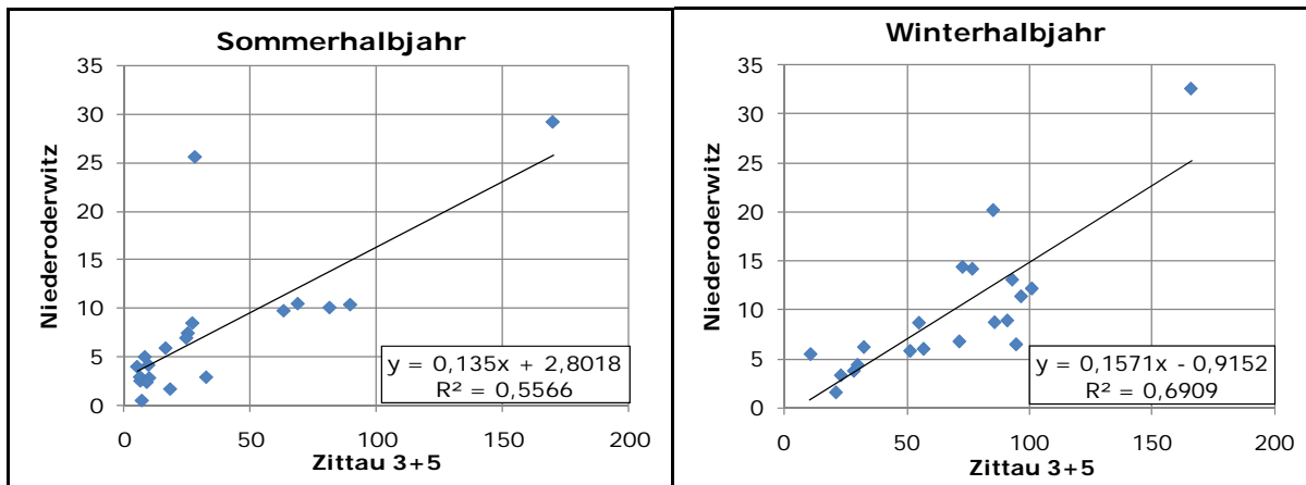
Abbildung 2: Regressionsbeziehungen zwischen den Höchstabflüssen an den Pegeln Niederoderwitz und Zittau 3+5
