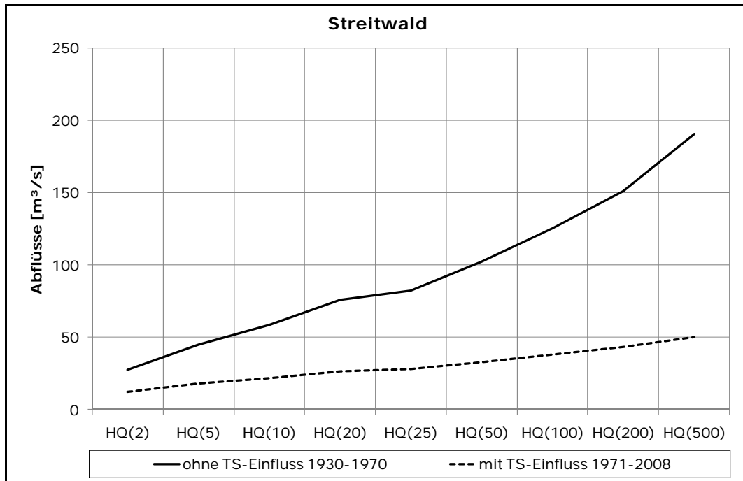
Abbildung 17: Extremwertstatistische Auswertung am Pegel Streitwald für die Zeitreihen ohne und mit Einfluss der Talsperre Schönbach
