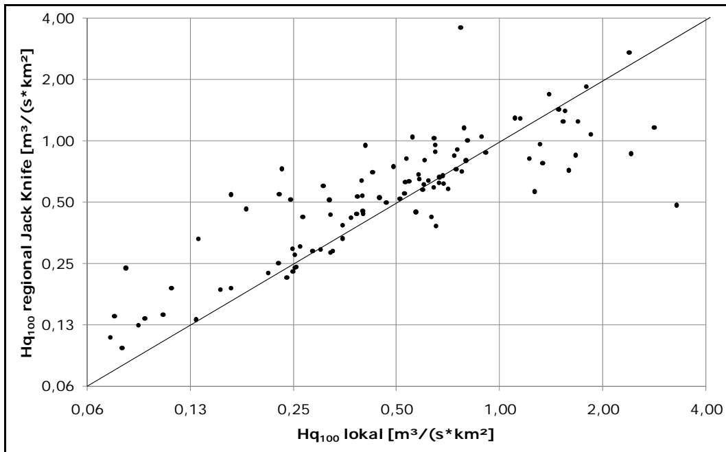
Abbildung 52: Gegenüberstellung der lokalen und der regionalisierten Abflusssspenden (Jack-Knife) für das Hq_{100} bei Methode 3
