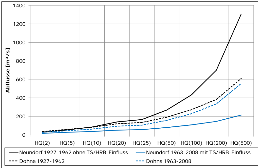
Abbildung 15: Extremwertstatistische Auswertung am Pegel Neundorf für die Zeitreihen Dohna und mit Einfluss von Stauanlagen und Vergleich mit dem Pegel Dohna/Müglitz
