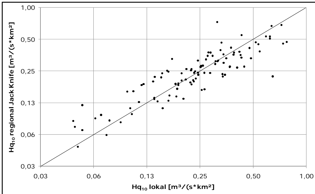
Abbildung 68: Gegenüberstellung der lokalen und der regionalisierten Abflussspenden (Jack-Knife) für das Hq_{10} bei Methode 5
