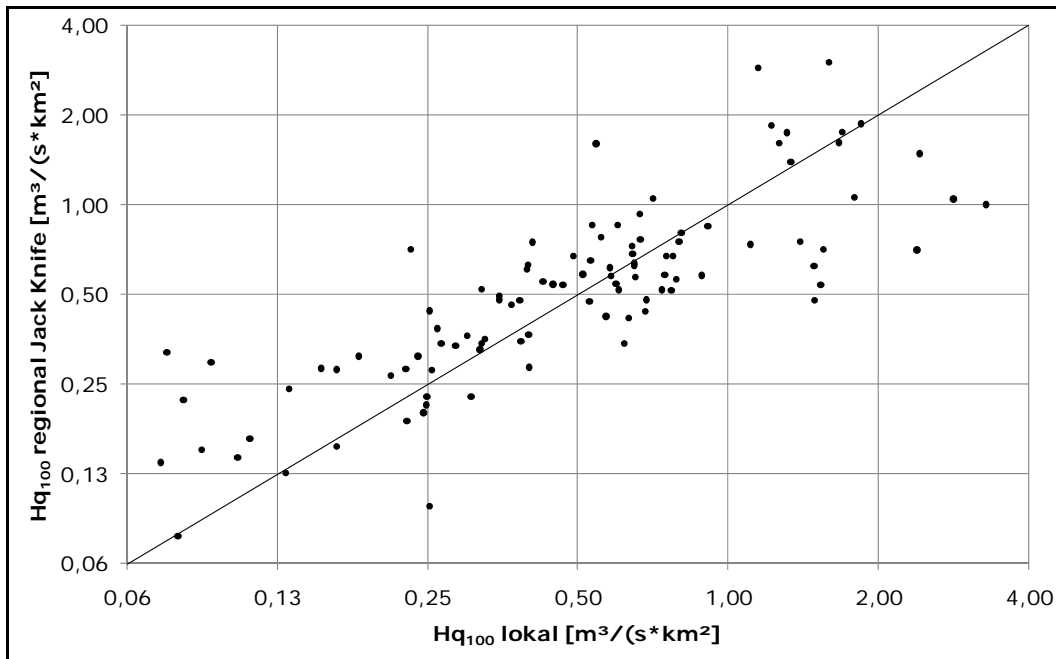
Abbildung 50: Gegenüberstellung der lokalen und der regionalisierten Abflusssspenden (Jack-Knife) für das H_{q100} bei Methode 2
