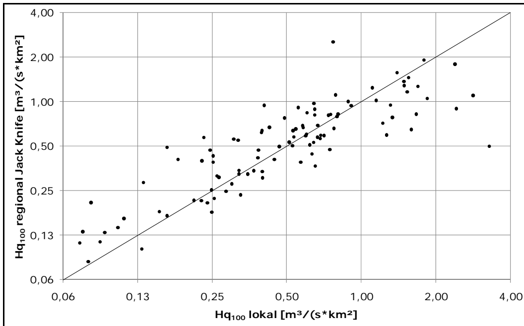
Abbildung 56: Gegenüberstellung der lokalen und der regionalisierten Abflussspenden (Jack-Knife) für das Hq_{100} bei Methode 5
