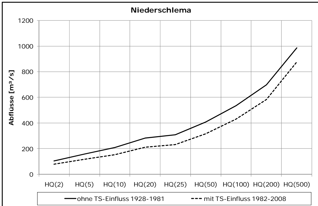
Abbildung 16: Extremwertstatistische Auswertung am Pegel Niederschlema für die Zeitreihen ohne und mit Einfluss der Talsperre Eibenstock
