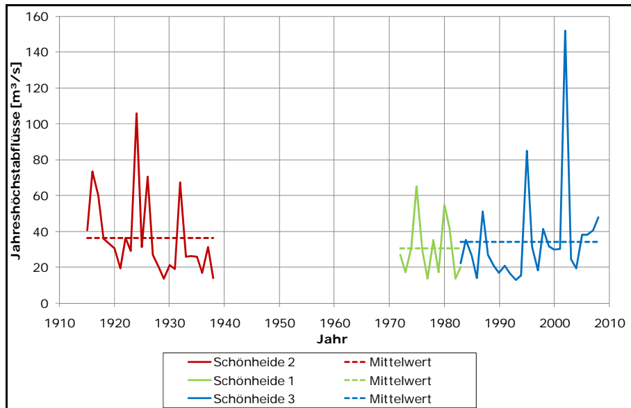
Abbildung 9: Jahreshöchstabflüsse der Pegel Schönheide 3 (PKZ 56201.2), Schönheide 2 (PKZ 56202.0) und Schönheide 1 (PKZ 56201.1) an der Zwickauer Mulde
