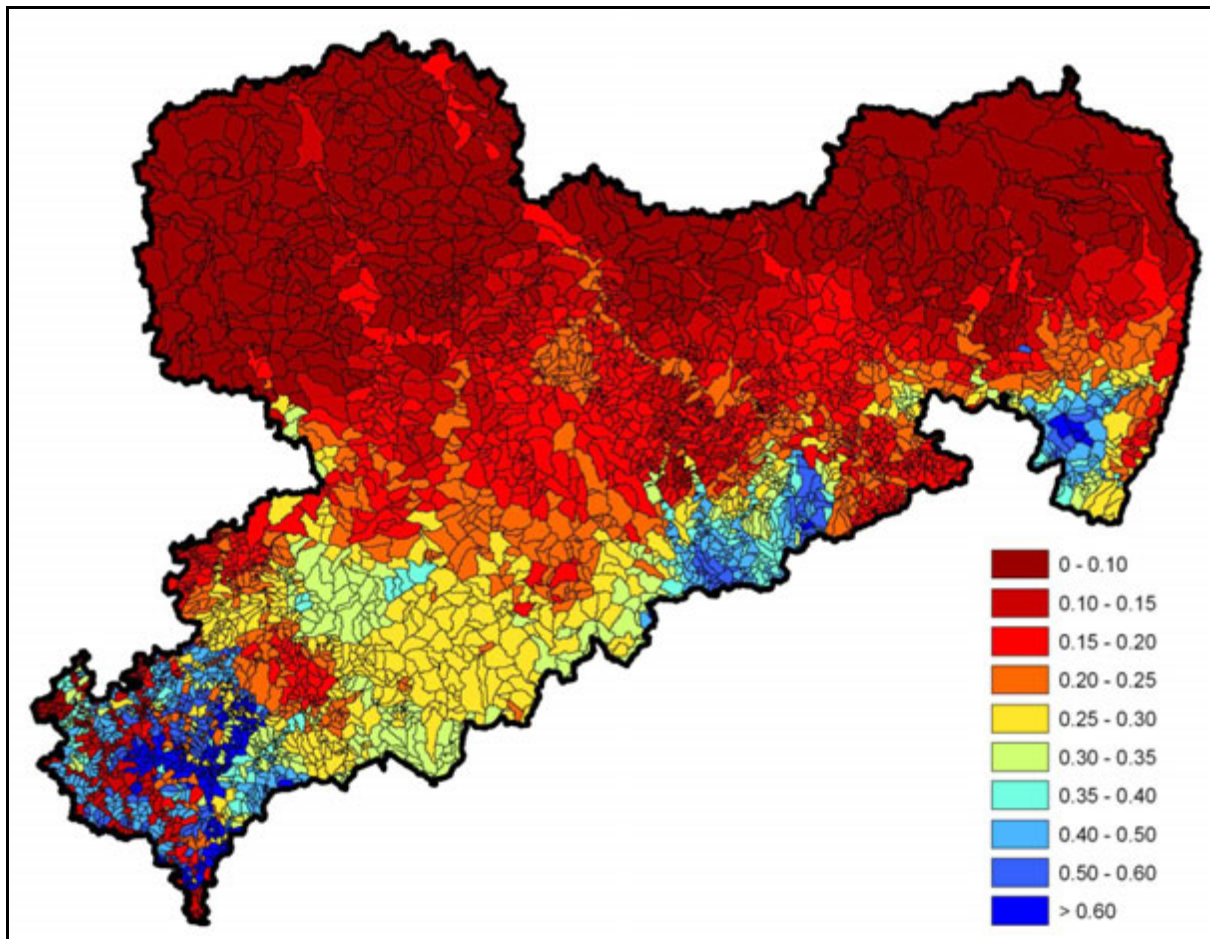
Abbildung 59: Hq 10 [m 3 /(s*km 2 )] ermittelt mit Top-Kriging – Methode 1
