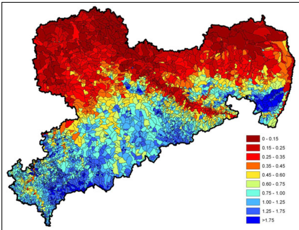
Abbildung 53: Hq_{100} [ m^3/(s \cdot km^2) ] ermittelt mit Index-Flood-Methode (AEV Parameter aus saisonaler HQ-Statistik), - Methode 4
