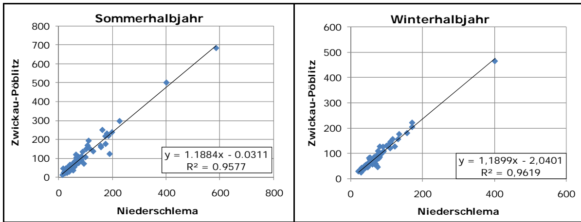
Abbildung 4: Regressionsbeziehungen zwischen den Höchstabflüssen an den Pegeln Zwickau-Pöblitz und Niederschlema
