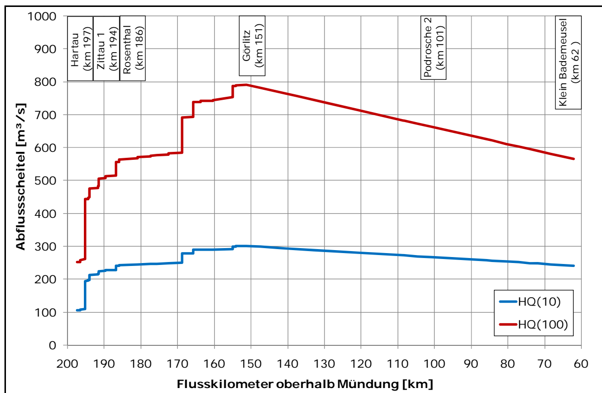
Abbildung 43: Abflusslängsschnitte der Lausitzer Neiße für das HQ 10 und HQ 100
