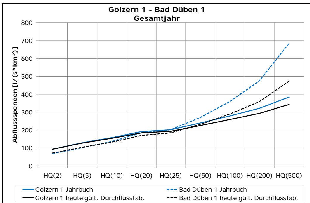
Abbildung 11: Vergleich der Hq_T der Pegel Golzern 1 und Bad Düben 1, wenn ausgewählte Extremabflüsse („Jahrbuchwerte“) durch Abflüsse gemäß den aktuellen W-Q-Beziehungen ersetzt werden
