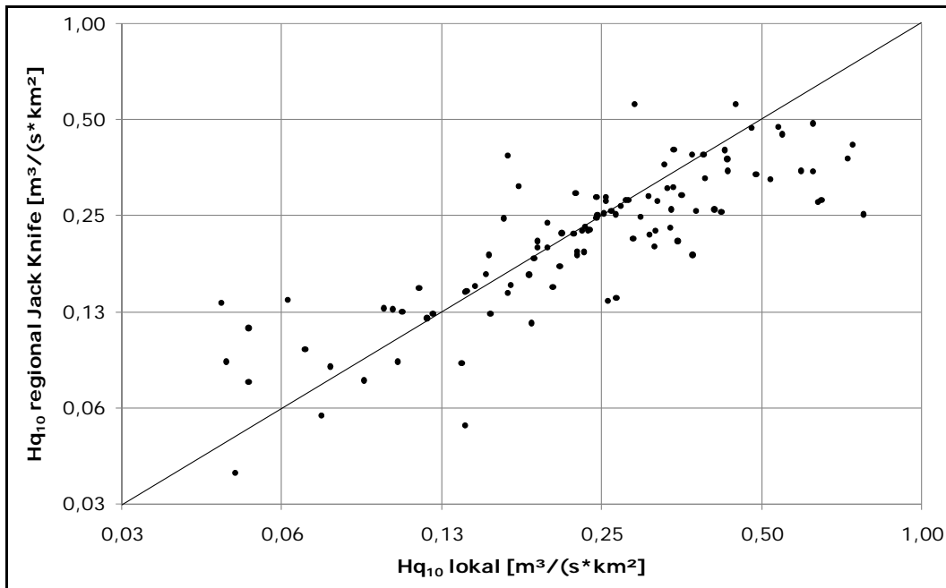
Abbildung 60: Gegenüberstellung der lokalen und der regionalisierten Abflussspenden (Jack-Knife) für das Hq 10 bei Methode 1
