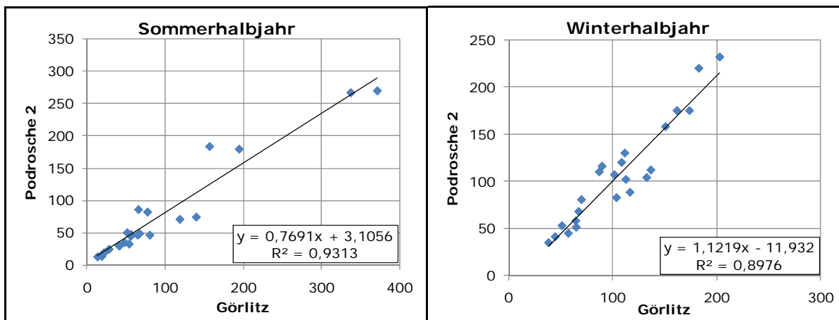
Abbildung 3: Regressionsbeziehungen zwischen den Höchstabflüssen an den Pegeln Podrosche 2 und Görlitz
