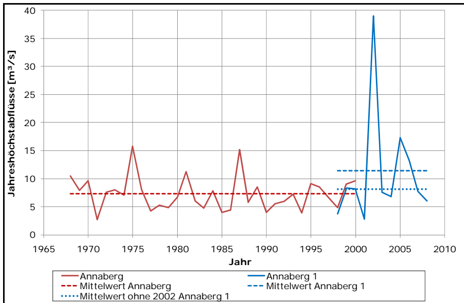
Abbildung 7: Jahreshöchstabflüsse der Pegel Annaberg 1 (PKZ 56759.0) und Annaberg (PKZ 56760.0) an der Sehma
