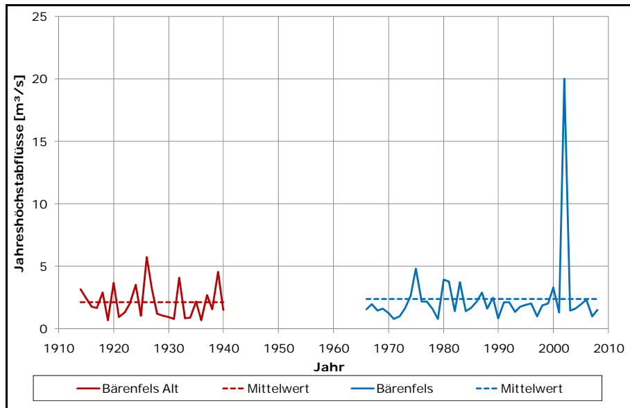
Abbildung 5: Jahreshöchstabflüsse der Pegel Bärenfels (PKZ 55151.0) und Bärenfels „Alt“ am Pöbelbach
