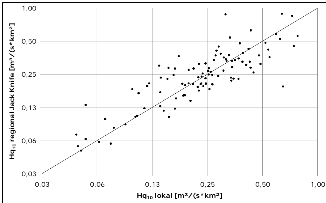
Abbildung 66: Gegenüberstellung der lokalen und der regionalisierten Abflussspenden (Jack-Knife) für das H_{q10} bei Methode 4
