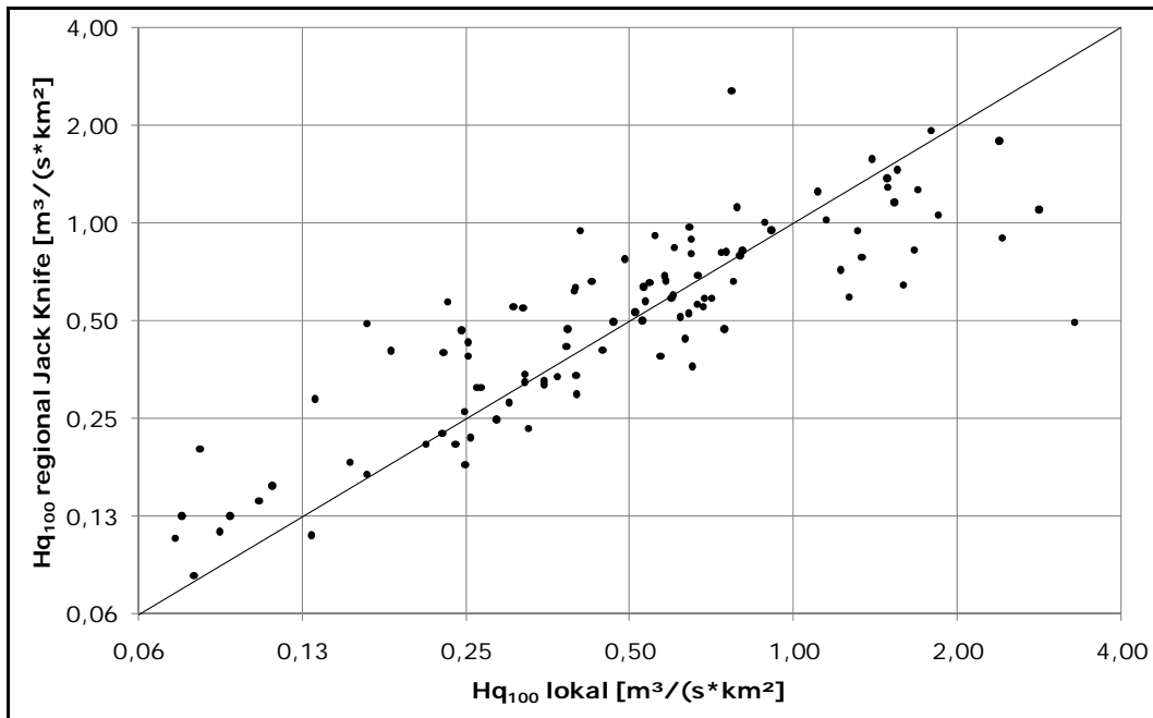
Abbildung 58: Gegenüberstellung der lokalen und der regionalisierten Abflussspenden (Jack-Knife) für das Hq 100 bei Methode 6
