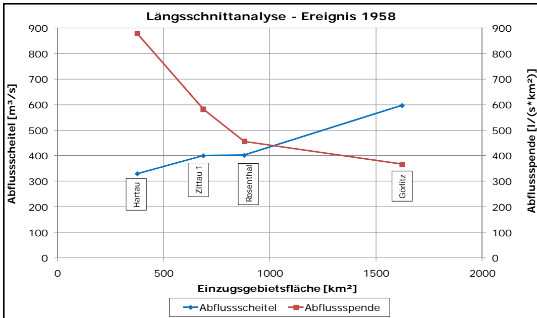
Abbildung 12: Beispiel für eine Längsschnittanalyse (Plausibilisierung des Hochwassers 1958 am Pegel Hartau/Lausitzer Neiße)
