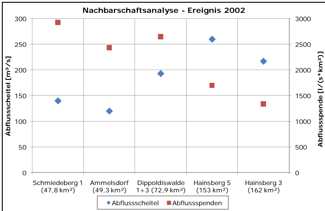
Abbildung 13: Beispiel für eine Nachbarschaftsanalyse (gegenseitige Plausibilisierung des Hochwassers 2002 an allen aufgeführten Pegeln)
