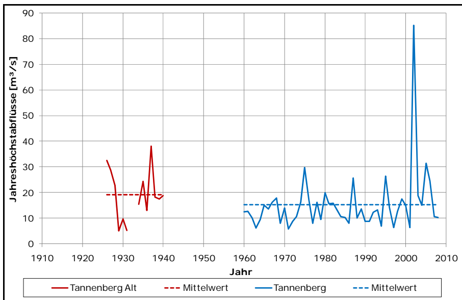
Abbildung 8: Jahreshöchstabflüsse der Pegel Tannenberg (PKZ 56740.0) und Tannenberg „Alt“ an der Zschopau
