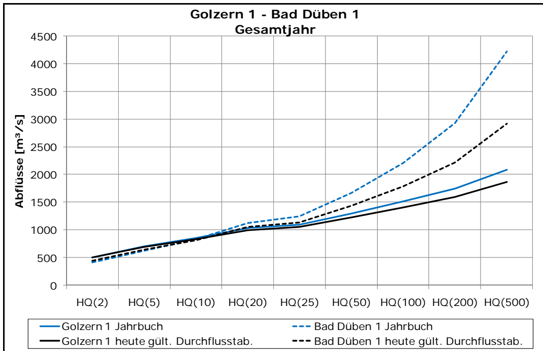
Abbildung 10: Vergleich der HQ_T der Pegel Golzern 1 und Bad Düben 1, wenn ausgewählte Extremabflüsse („Jahrbuchwerte“) durch Abflüsse gemäß der aktuellen W-Q-Beziehungen ersetzt werden
