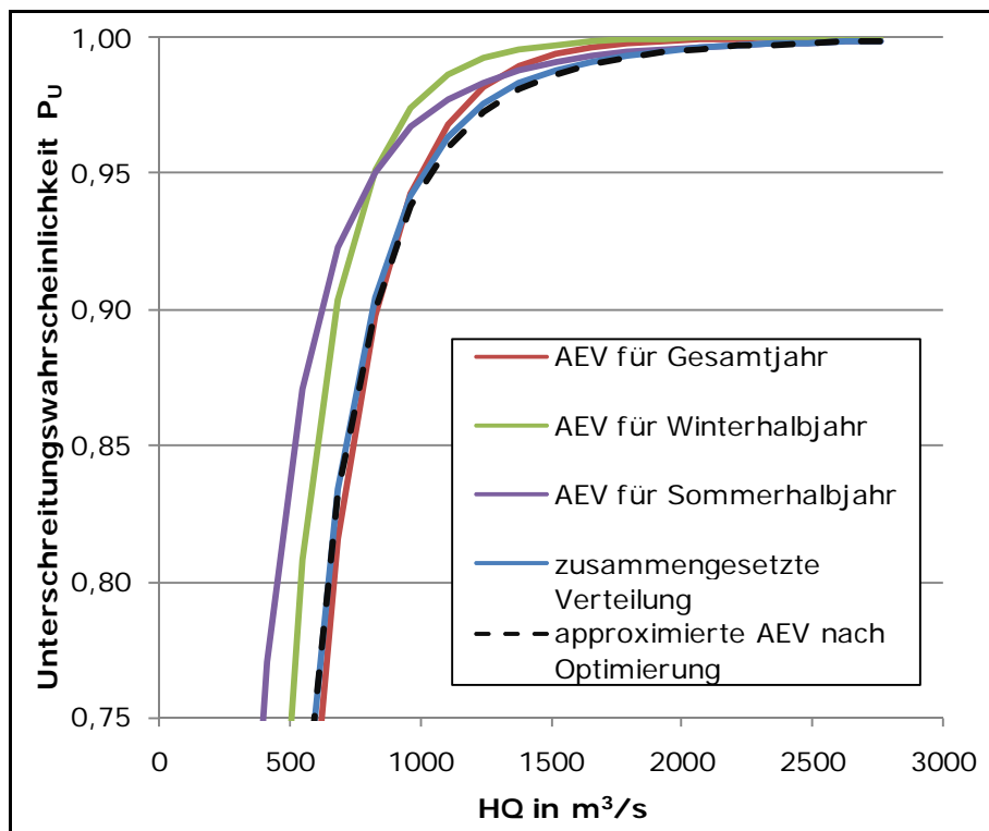
Abbildung 18: Approximation einer Allgemeinen Extremwertverteilung an die zusammengesetzte Verteilung am Beispiel des Pegels Golzern 1/Mulde
