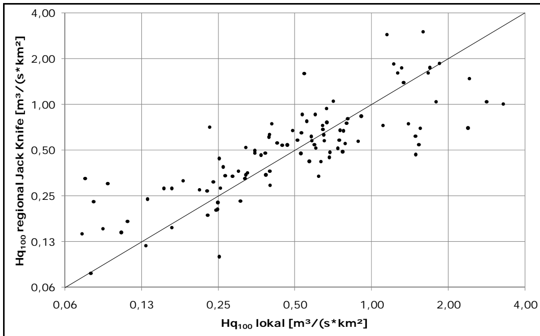
Abbildung 48: Gegenüberstellung der lokalen und der regionalisierten Abflusspenden (Jack-Knife) für das Hq_{100} bei Methode 1
