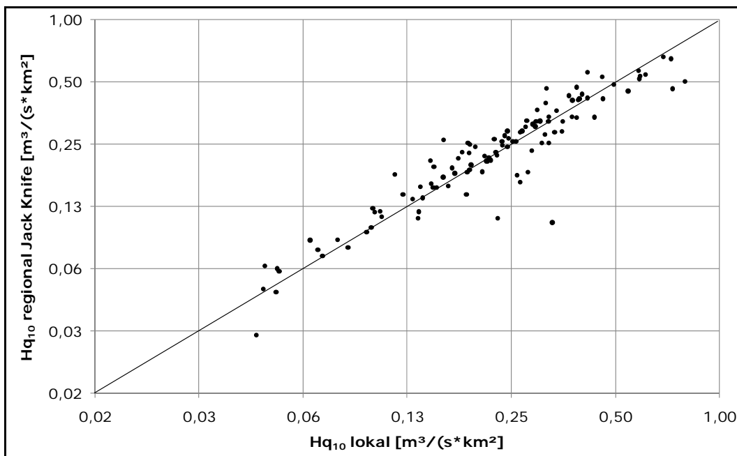
Abbildung 75: Gegenüberstellung der lokalen und der regionalisierten Abflussspenden (Jack-Knife) für das Hq_{10} bei der erweiterten Methode 6
