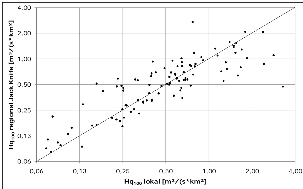
Abbildung 54: Gegenüberstellung der lokalen und der regionalisierten Abflussspenden (Jack-Knife) für das H_{q100} bei Methode 4
