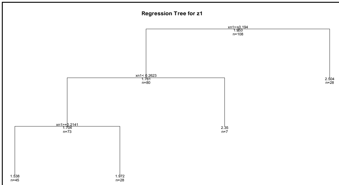
Abbildung 31: Regressionsbaum für Xn1, 4 Gruppen
