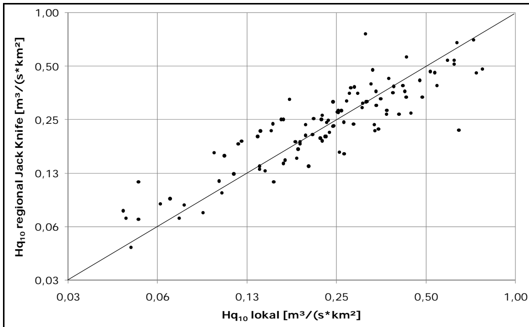
Abbildung 70: Gegenüberstellung der lokalen und der regionalisierten Abflussspenden (Jack-Knife) für das Hq 10 bei Methode 6
