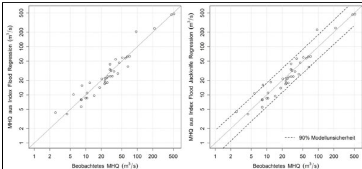
Abbildung 34: Gegenüberstellung der beobachteten MHQ gegen die anhand des Index-Flood/Regression (links) und des Index-Flood/Regression Jack-Knife (rechts) ermittelten MHQ für Region 1
