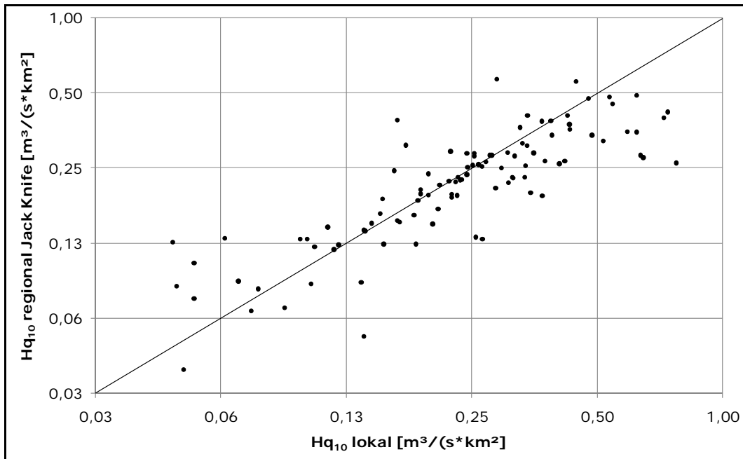
Abbildung 62: Gegenüberstellung der lokalen und der regionalisierten Abflussspenden (Jack-Knife) für das Hq 10 bei Methode 2
