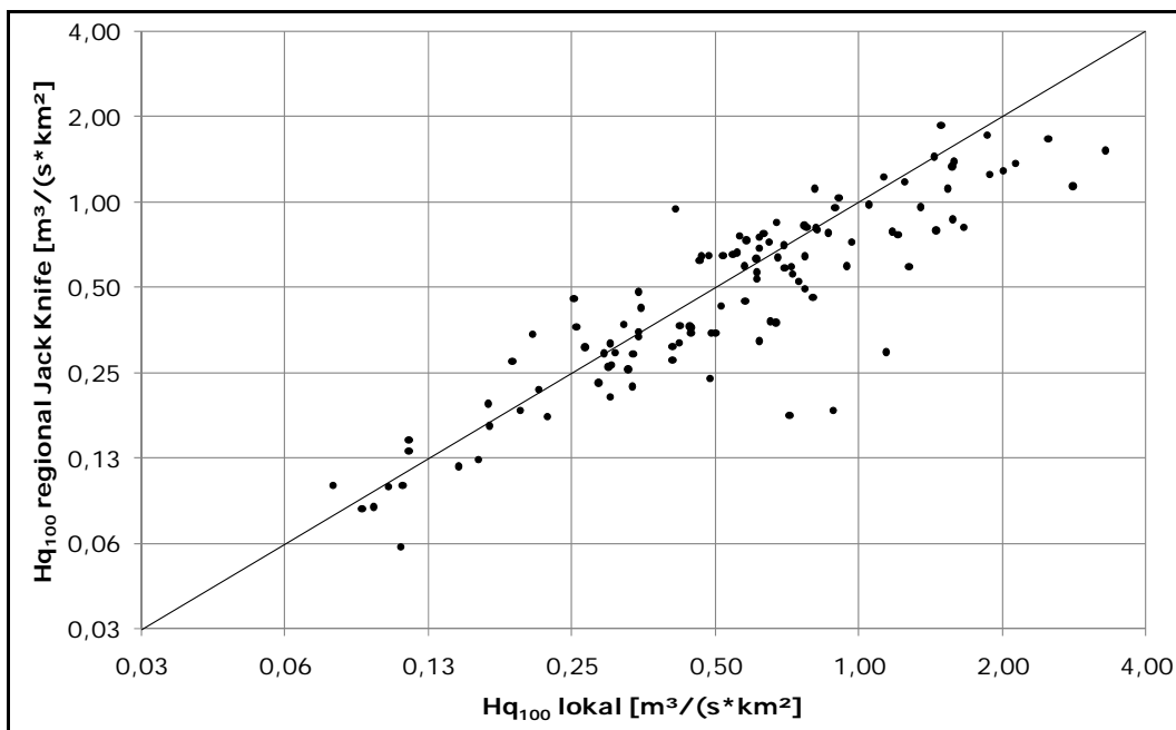
Abbildung 73: Gegenüberstellung der lokalen und der regionalisierten Abflussspenden (Jack-Knife) für das Hq_{100} bei der erweiterten Methode 6
