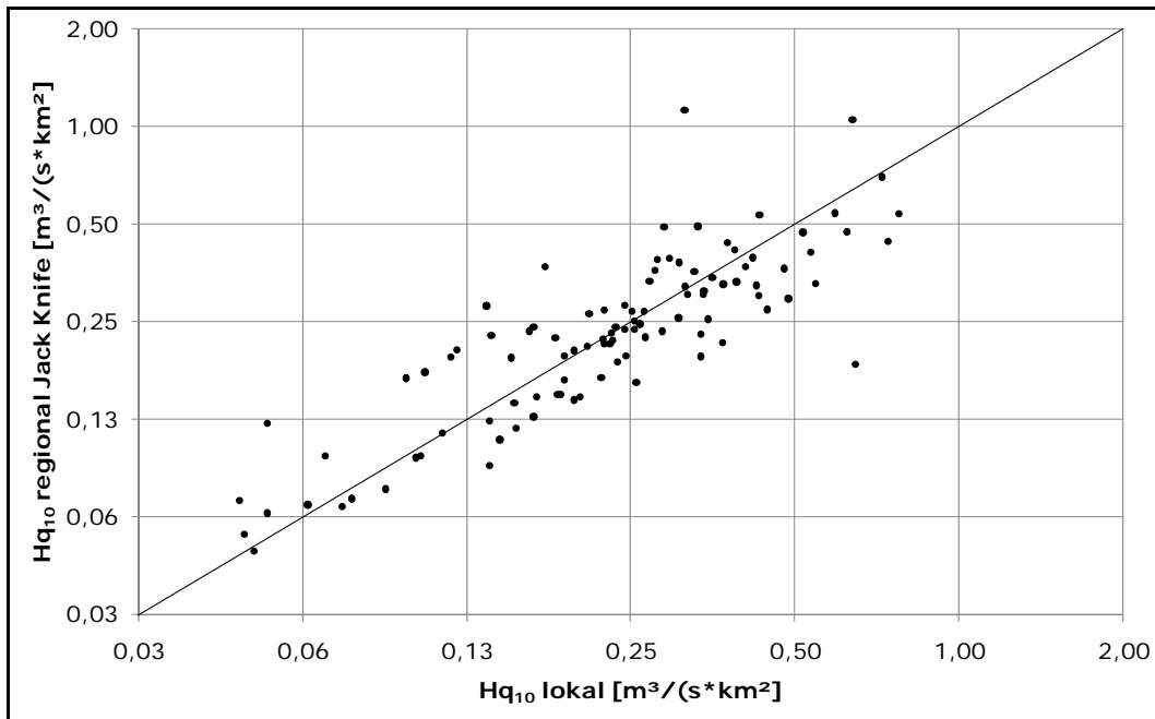
Abbildung 64: Gegenüberstellung der lokalen und der regionalisierten Abflussspenden (Jack-Knife) für das Hq_{10} bei Methode 3
