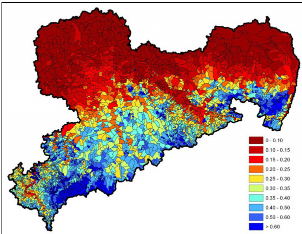
Abbildung 63: Hq 10 [m³/(s*km²)] ermittelt mit Index-Flood-Methode (AEV Parameter aus HQ Reihe) – Methode 3
