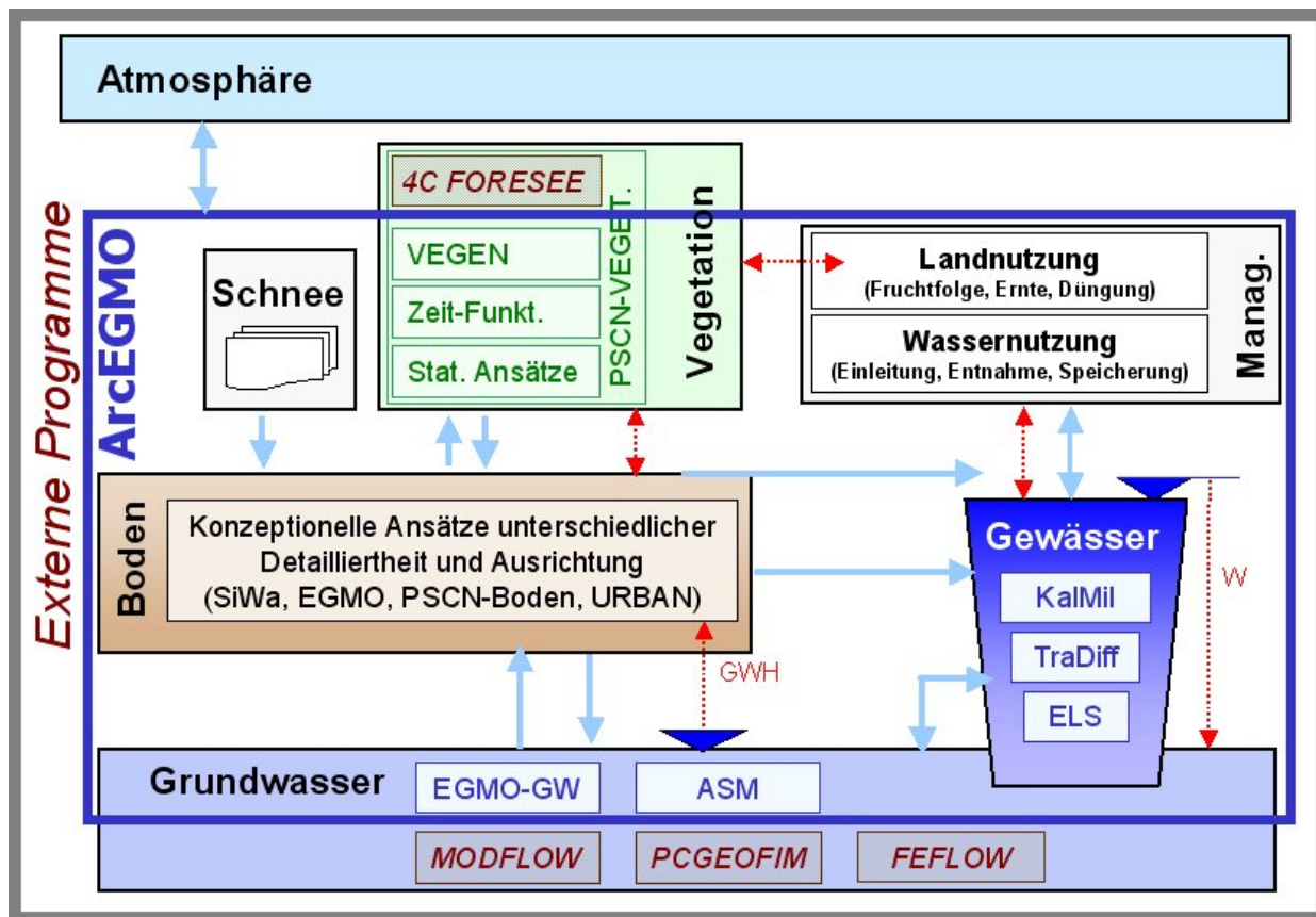
Abbildung 2: Modellebenen des Modellierungssystems ArcEGMO
