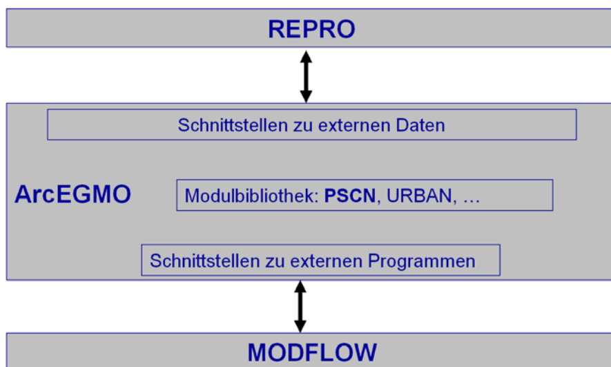
Abbildung 8: Funktionsbild ReArMo
