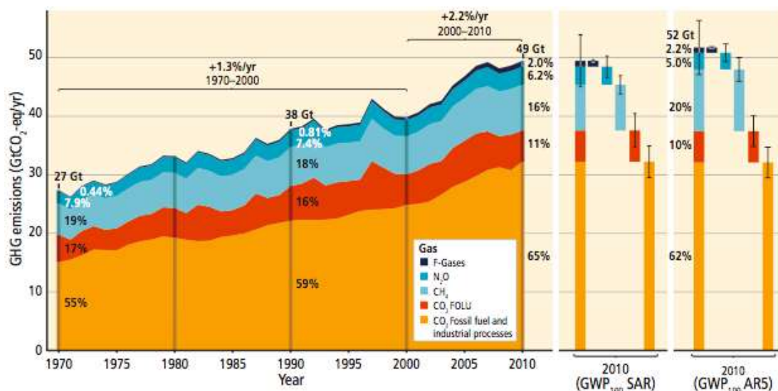
Figura 2: Total anual de Emissões antropogênicas de GEE por gases entre 1970 e 2010. Fonte: IPCC, 2014.
