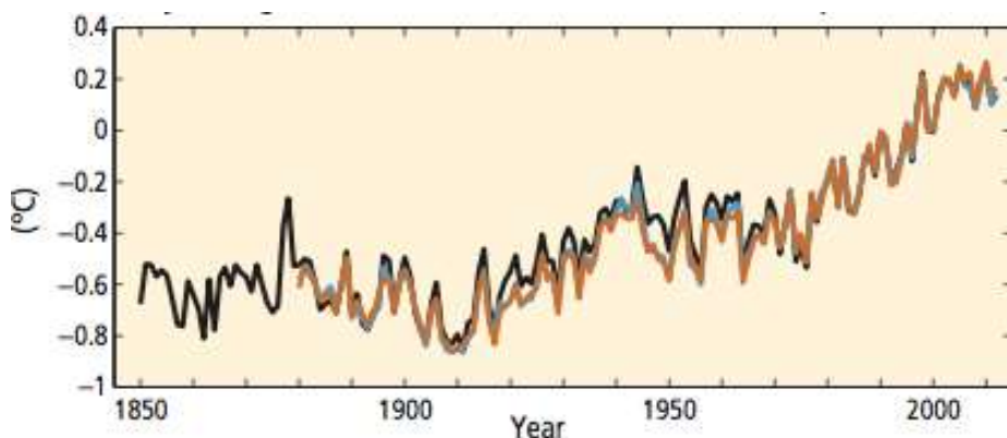
Figura 1: Temperatura média global combinada das superfícies terrestres e oceânicas. Fonte: IPCC, 2014.
