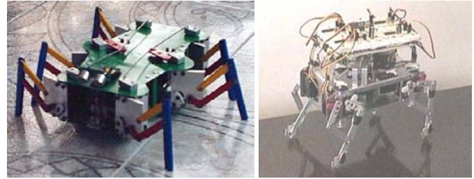
(a) (b) Figura 2. Robots con sistemas de locomoción por patas (a) Hexápodo (b) Cuadrúpedo.
