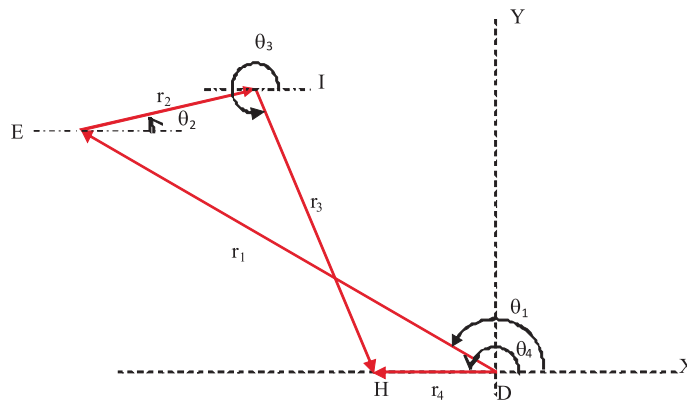
Figura 4. Mecanismo cruzado de cuatro barras
