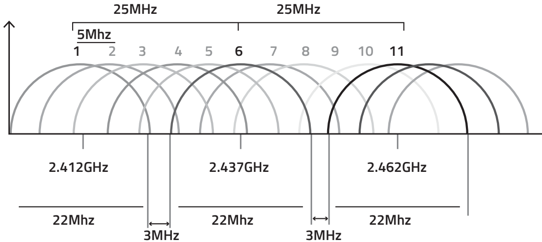
Figura 2. Canales No interferibles y anchos de banda
