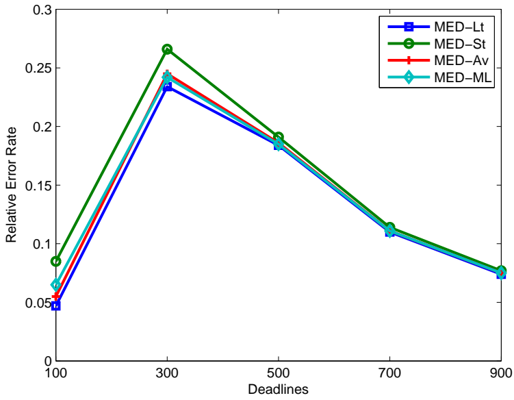
Fig. 6. Relative error rate of the MED predictor
