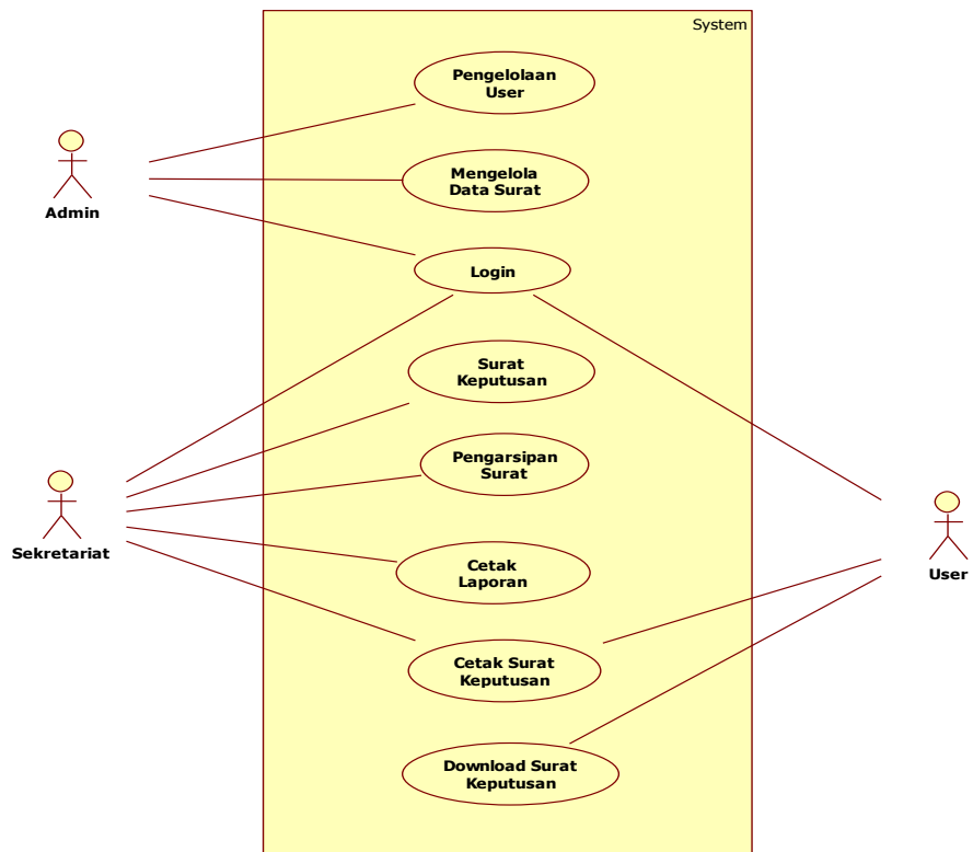
Gambar 4. 1 Use Case Diagram yang di usulkan
