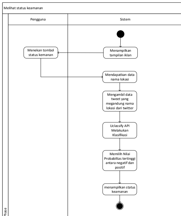
Gambar 12. Acitivity Diagram Lihat Status Keamanan
