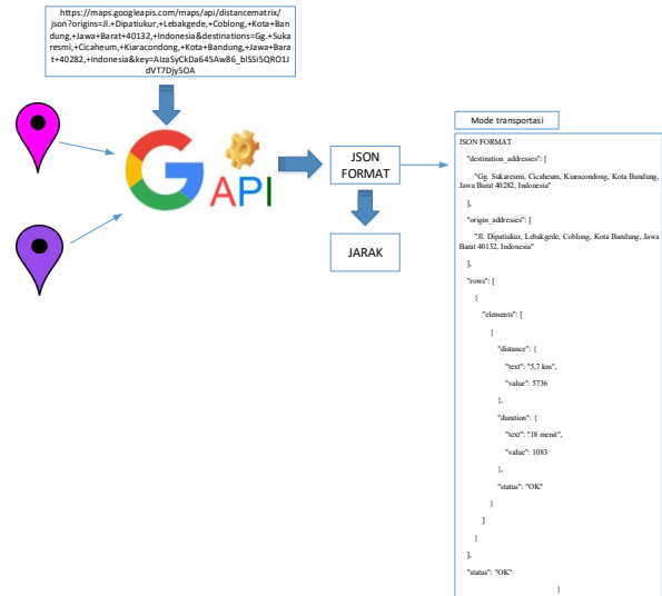
Gambar 9. Analisis Mendapatkan Jarak
