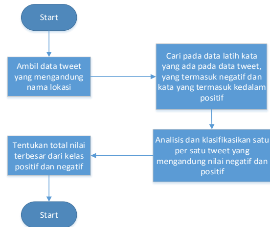
Gambar 8. Analisis Prosedur Aplikasi
