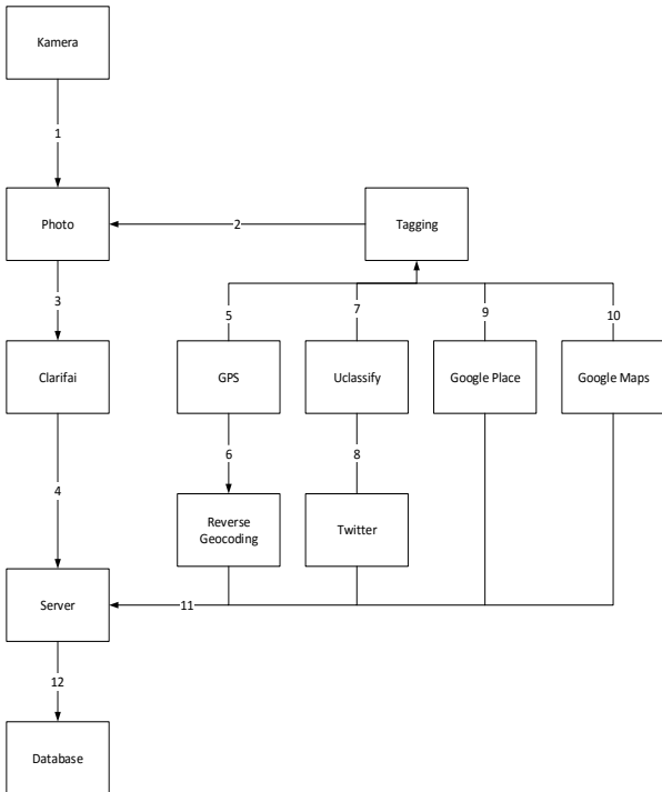
Gambar 5. Analisis Prosedur Aplikasi
