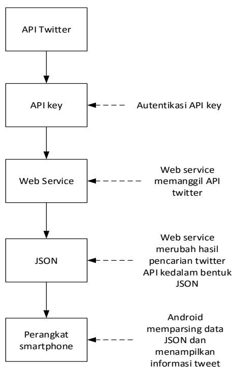
Gambar 7. Analisis Prosedur Aplikasi
