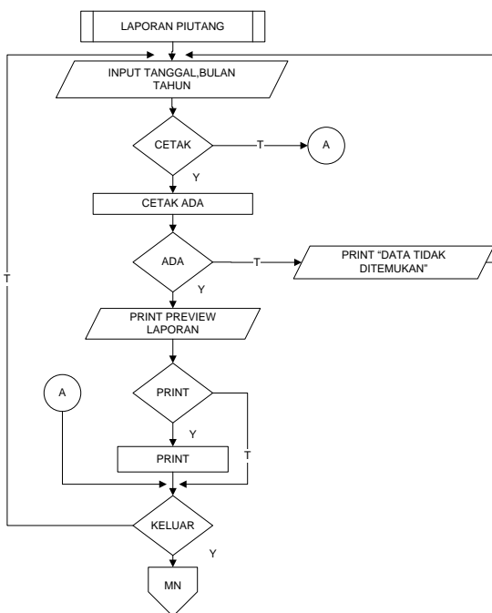
Gambar 29. Lanjutan Flowchart Form Laporan
