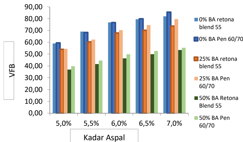
Gambar 19. Perbandingan aspal retona blend 55 dan aspal pen 60/70
