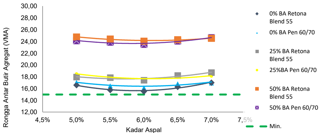
Gambar 6. Grafik hubungan kadar aspal dengan VMA menggunakan aspal retona blend 55
