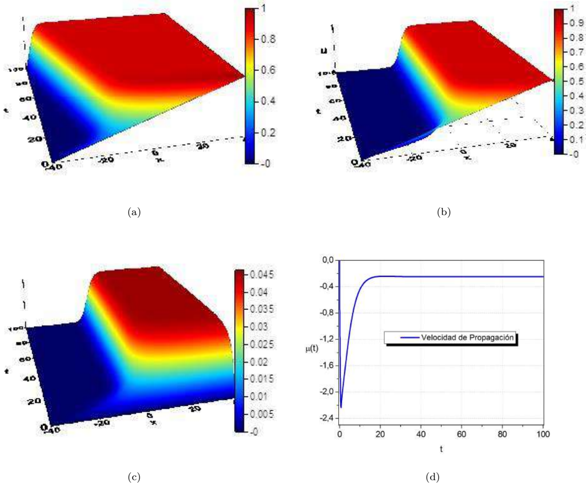
FIGURA 4.1. Perfil espacio-temporal de la frente viajera, componente u , para el sistema FHN, sistema(2.1), en coordenadas locales (a), perfil de la frente viajera en el sistema FHN, sistema (3.6), en coordenadas no locales para la componente u (b), componente w para el sistema FHN en coordenadas no locales, sistema (3.1)(c) y velocidad de propagación \mu (d).
