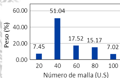
Figura 2. Distribución de tamaño de partículas retenidas en las mallas 20, 40, 50, 80, 100 de harina de papa.
