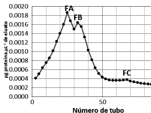
Figura 2. Cromatografía en columna con Sephadex G-100 desde EC del látex de Vasconcella candidans (A. Gray) A. DC 1864 (Mito): Columna 21,0 x 2,0 cm, buffer acetato 50 mM, pH 5,6; promedio de flujo: 1 \text{ mL}\cdot\text{min}^{-1} . Se muestra la concentración de proteína ( A_{280\text{nm}} ) de cada eluato.
