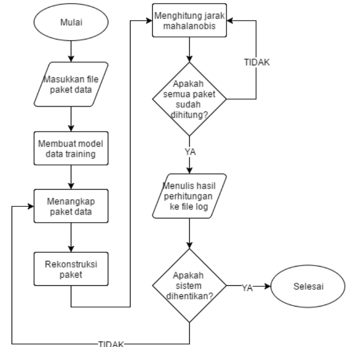
Gambar 1 Diagram alir kerja sistem secara umum
