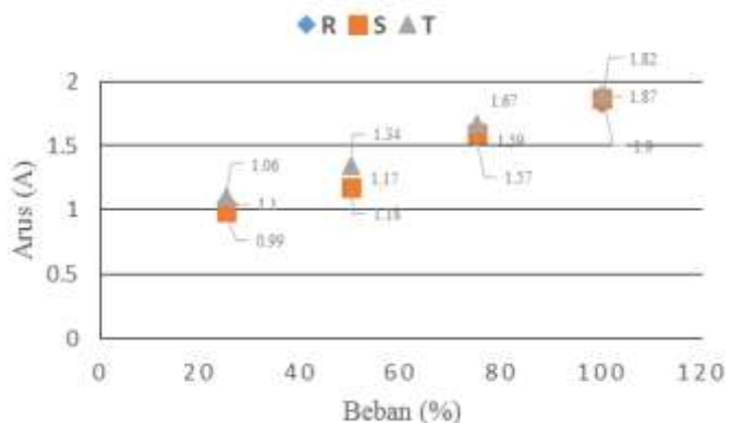
Gambar 9. Arus Pada Kondisi Short R-T Turn 1
