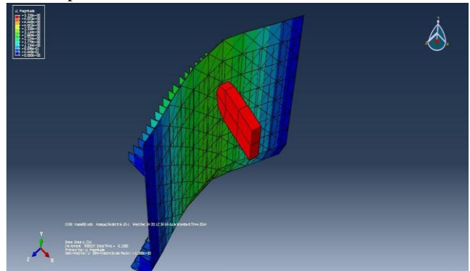
Gambar. 4. Pemodelan dengan dampak energi 725.89MJ
