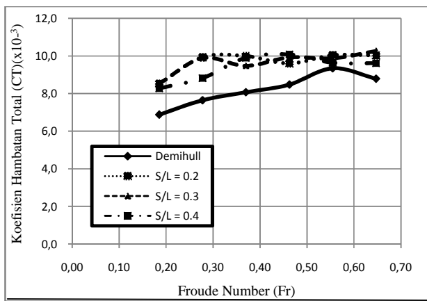
Gambar 6. Koefisien hambatan total melalui CFD.
