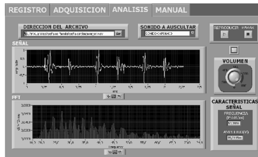
Fig 15. Etapa de Análisis
