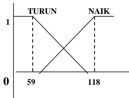
Gambar 3. Fungsi keanggotaan himpunan fuzzy TURUN dan NAIK dari variabel Permintaan
