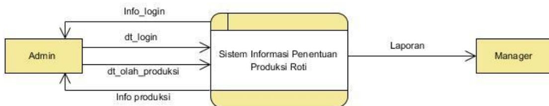
Gambar 7. Diagram Konteks Penentuan Produksi Roti
