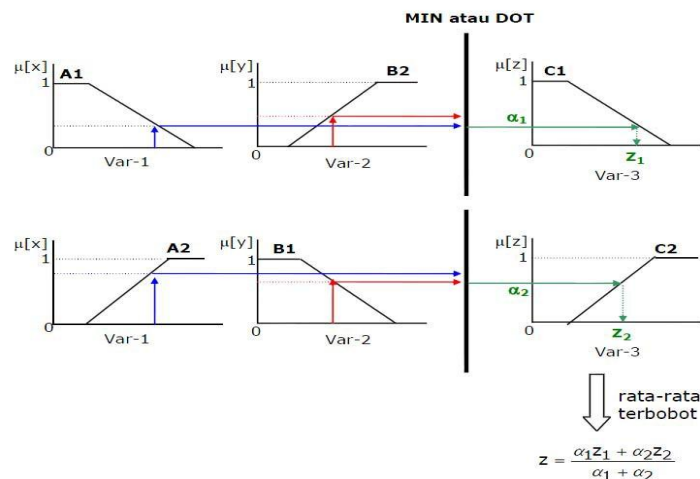
Gambar 1. Proses inferensi dengan menggunakan metode Tsukamoto
