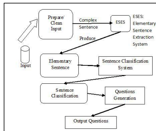
Gambar 5. Kerangka kerja AQG Ali dkk[6]
