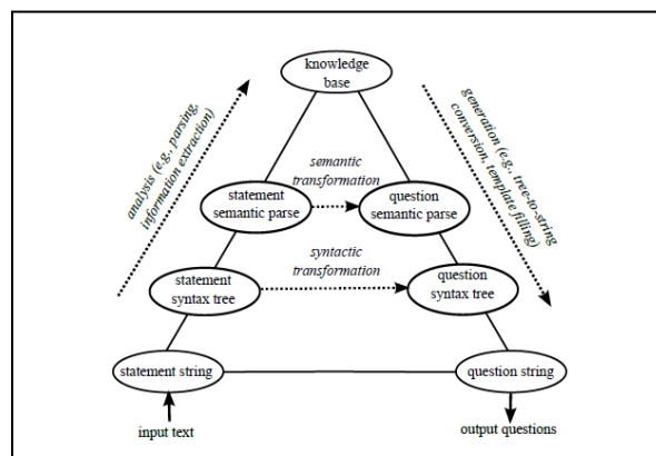
Gambar 4. Segitiga Vauquois[16]
