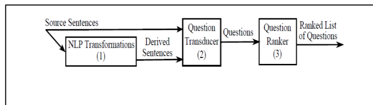
Gambar 4. Kerangka Kerja tiga tahap Heilman dan Smith[20]
