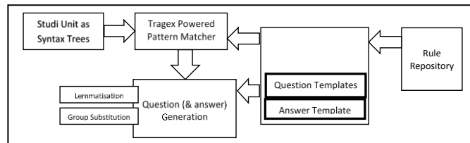
Gambar 3. Kerangka kerja Automated question generation (AQG) Bednarik dan Kovács[10].
