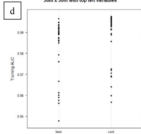
30mbest10 AUC 0.982
