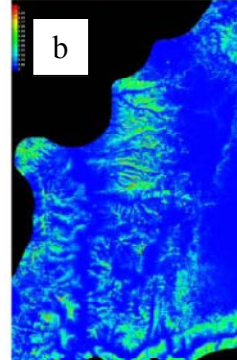
30mtrainbest4 AUC 0.938
