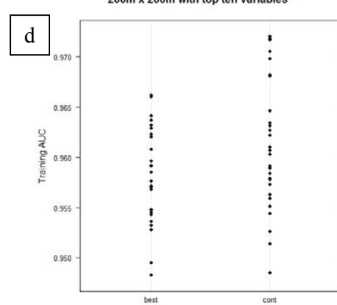
200mbest10 AUC 0.958
