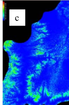
30mbest4 AUC 0.968
