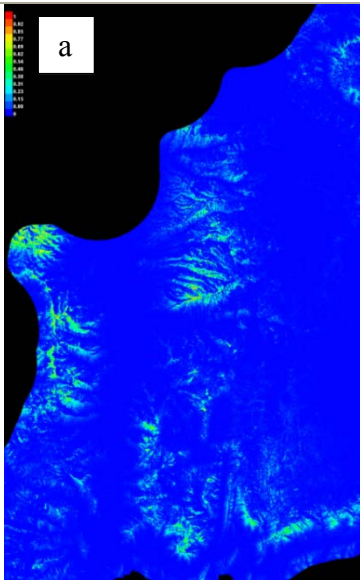
30mcontbest10 AUC 0.987
