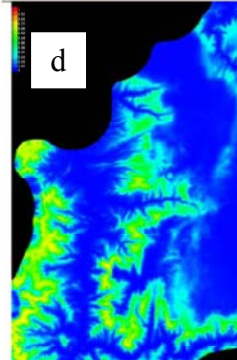
30maucbest4 AUC 0.929
