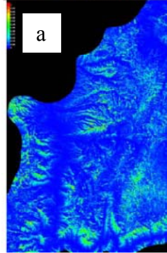
30mcontbest4 AUC 0.962
