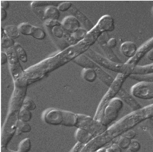
Nomarski
