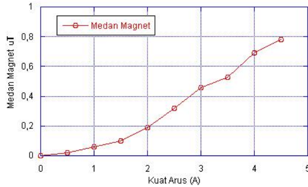
Gambar 3. Perubahan medan magnet terhadap kuat arus listrik
