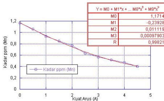
Gambar 7. Perubahan kadar ppm mangan (Mn) terhadap arus
