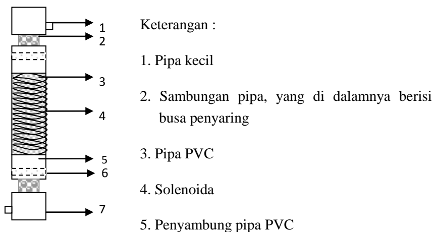
Gambar 2. Skema penyaring elektromagnetik
