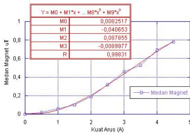
Gambar 4. Pendekatan kurva perubahan kuat arus
