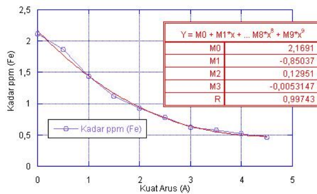
Gambar 6. Perubahan kadar ppm besi (Fe) terhadap arus
