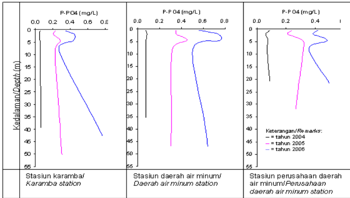
Gambar 11. Hubungan antara konsentrasi P-PO 4 (mg per l) dengan kedalaman (m) di stasiun pengamatan karamba, daerah air minum, dan perusahaan daerah air minum pada tahun 2004 (—), 2005 (—), dan 2006 (—).
