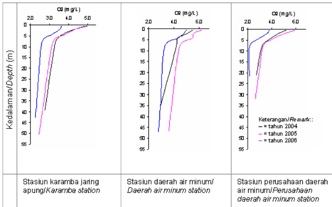
Gambar 4. Hubungan antara konsentrasi oksigen terlarut (mg per l) dengan kedalaman (m) di stasiun pengamatan karamba jaring apung, daerah air minum, dan perusahaan daerah air minum pada tahun 2004 (—), 2005 (—), dan 2006 (—).
