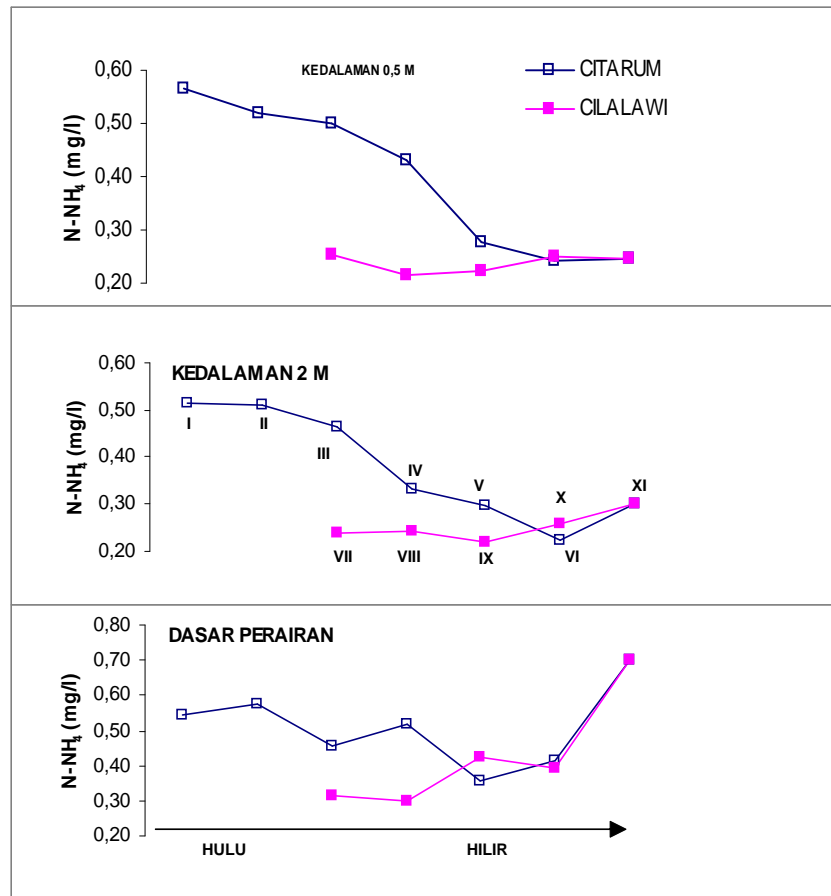
Gambar 9. Rata-rata N-NH 4 (mg per l) pada kedalaman permukaan (0,5 m), 2, m dan dasar perairan menurut stasiun pengamatan alur Sungai Citarum dan Cilalawi.
