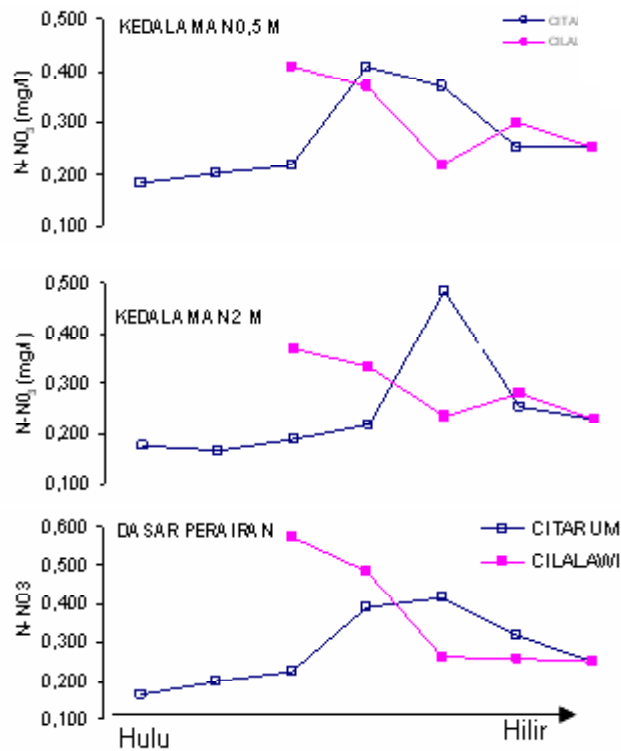
Gambar 7. Rata-rata nitrat (mg per l) pada kedalaman permukaan (0,5 m), 2 m dan dasar perairan menurut stasiun pengamatan alur Sungai Citarum dan Cilalawi.
