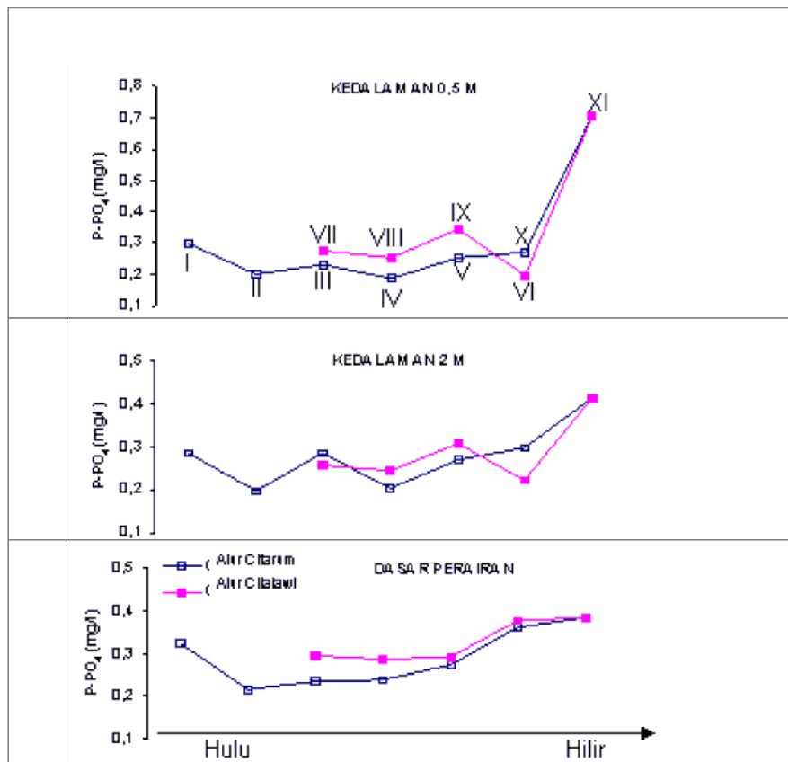
Gambar 10b. Rata-rata P-PO 4 (mg per l) pada kedalaman permukaan (0,5 m), 2 m dan dasar perairan menurut stasiun pengamatan alur Sungai Citarum dan Cilalawi. Figure 10b. Average of P-PO 4 (mg per l) in surface (0,5 m), 2 m and bottom waters by observation station groove of Citarum and Cilalawi River.
