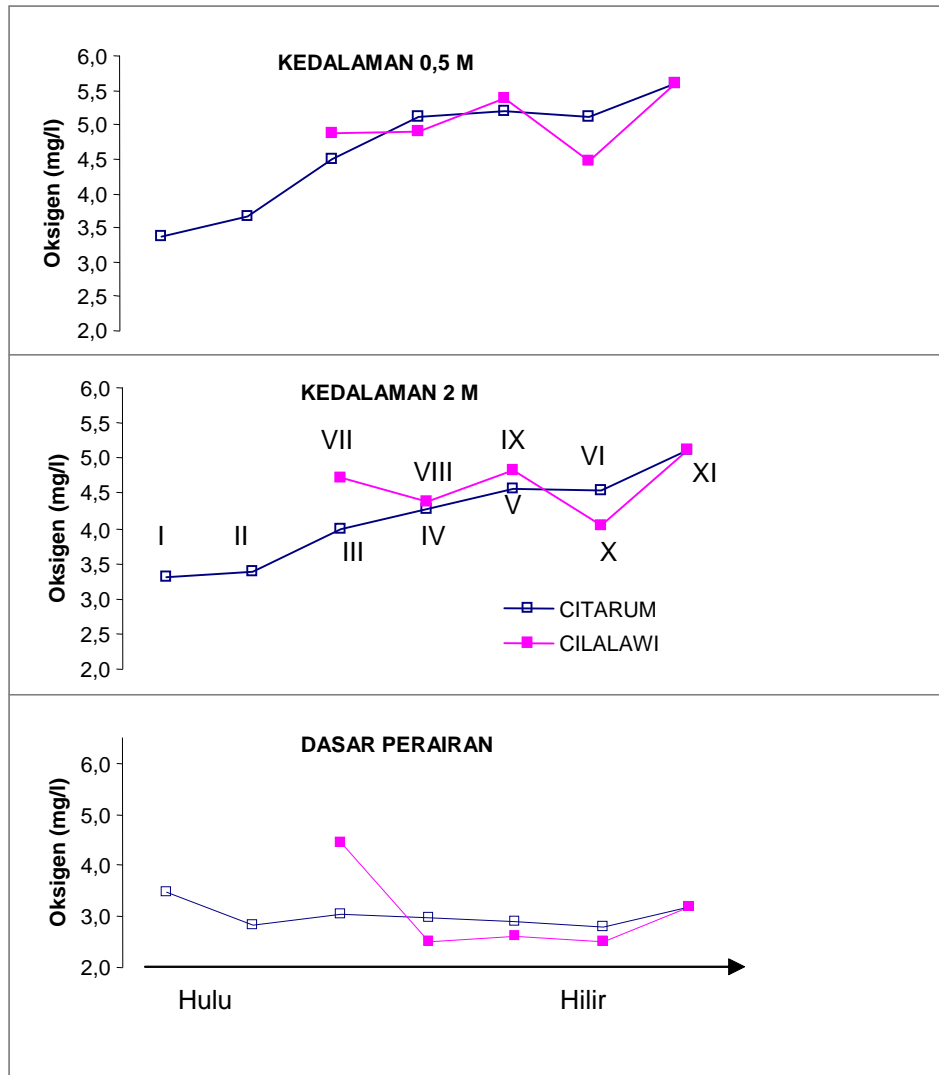
Gambar 3. Rata-rata oksigen terlarut pada kedalaman permukaan (0,5 m), 2 m dan dasar perairan menurut stasiun pengamatan alur Sungai Citarum dan Sungai Cilalawi.
