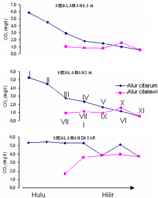
Gambar 6. Rata-rata Karbon dioksida (mg per l) pada kedalaman permukaan (0,5 m), 2 m, dan dasar perairan menurut stasiun pengamatan alur Sungai Citarum dan Cilalawi.
