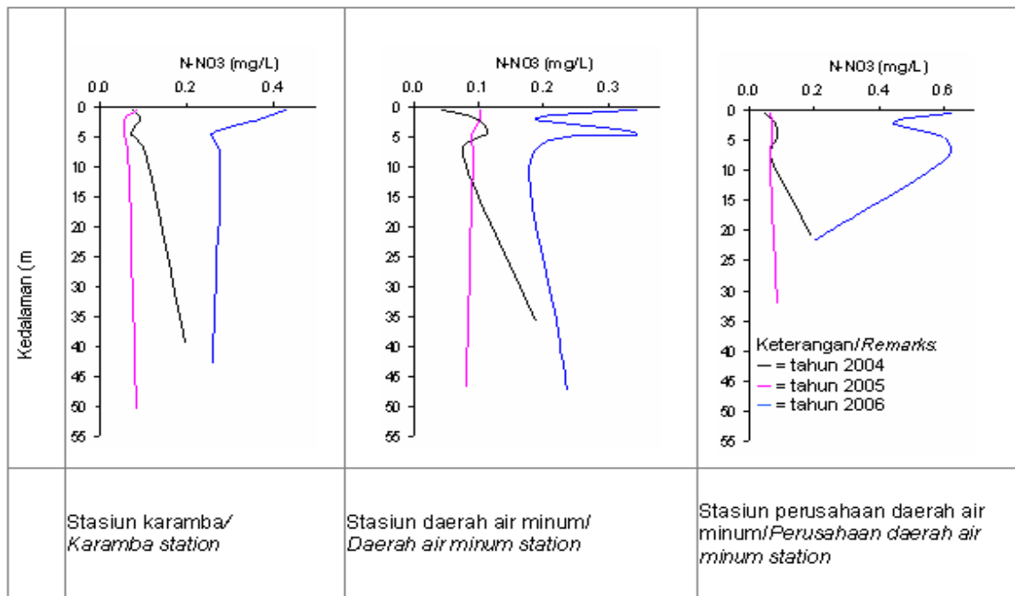
Gambar 8. Hubungan antara konsentrasi N-NO_3 (mg per l) dengan kedalaman (m) di stasiun pengamatan karamba, daerah air minum, dan perusahaan daerah air minum pada tahun 2004 (—), 2005 (—), dan 2006 (—).
