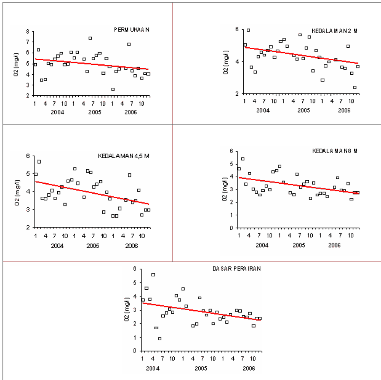
Gambar 5. Rata-rata oksigen (mg per l) terlarut pada kedalaman permukaan (0,5 m), 2; 4,5; dan 8 m dan dasar perairan menurut waktu pengamatan.
